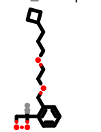
PhEthOH_3641.pdb
