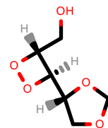
PhEthOH_454.pdb
