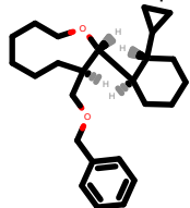
PhEthOH_3333.pdb
