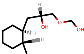
PhEthOH_360.pdb
