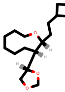
PhEthOH_3521.pdb
