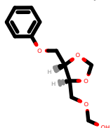
PhEthOH_508.pdb
