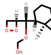
PhEthOH_367.pdb
