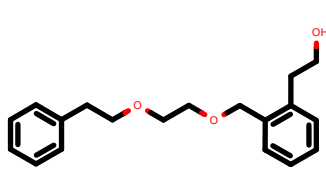
PhEthOH_1021.pdb
