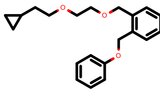
PhEthOH_3154.pdb
