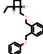
PhEthOH_1554.pdb
