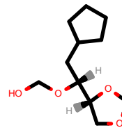
PhEthOH_3859.pdb
