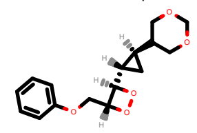
PhEthOH_4921.pdb
