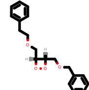
PhEthOH_1021.pdb
