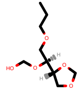
PhEthOH_159.pdb
