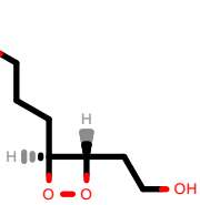
PhEthOH_1821.pdb
