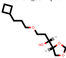
PhEthOH_3644.pdb
