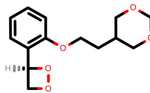
PhEthOH_4690.pdb
