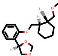
PhEthOH_2088.pdb
