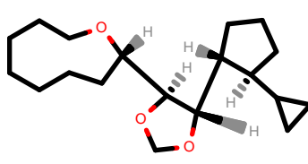
PhEthOH_3321.pdb
