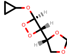
PhEthOH_3062.pdb
