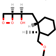
PhEthOH_2084.pdb
