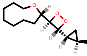
PhEthOH_254.pdb
