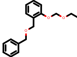
PhEthOH_1354.pdb
