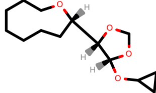
PhEthOH_3069.pdb
