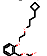
PhEthOH_3634.pdb
