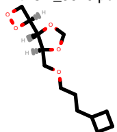
PhEthOH_3644.pdb
