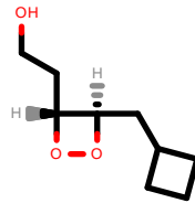
PhEthOH_3421.pdb
