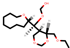
PhEthOH_2559.pdb
