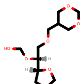
PhEthOH_4821.pdb
