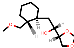
PhEthOH_2090.pdb
