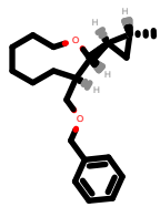
PhEthOH_221.pdb
