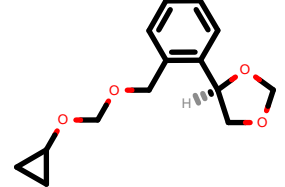
PhEthOH_3059.pdb
