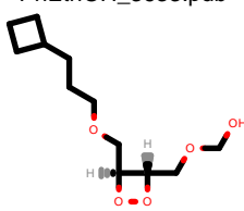
PhEthOH_3637.pdb
