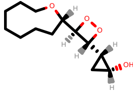
PhEthOH_670.pdb
