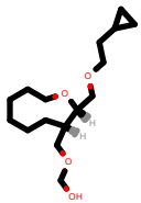
PhEthOH_3177.pdb
