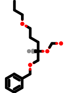
PhEthOH_2654.pdb
