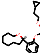
PhEthOH_3190.pdb
