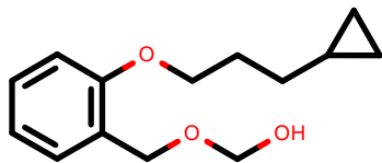
PhEthOH_3088.pdb
