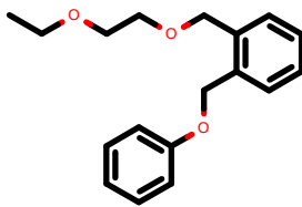
PhEthOH_84.pdb
