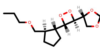
PhEthOH_2890.pdb
