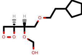
PhEthOH_4021.pdb
