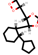
PhEthOH_4190.pdb
