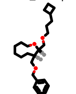
PhEthOH_3627.pdb
