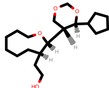
PhEthOH_4221.pdb
