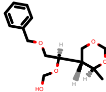
PhEthOH_390.pdb
