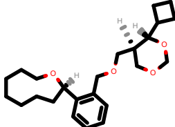
PhEthOH_3821.pdb
