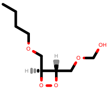
PhEthOH_189.pdb
