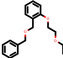
PhEthOH_90.pdb
