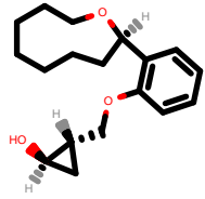
PhEthOH_670.pdb
