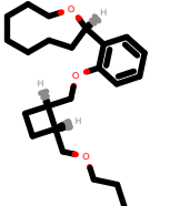
PhEthOH_2854.pdb
