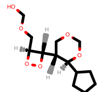
PhEthOH_4221.pdb
