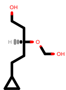
PhEthOH_3084.pdb
