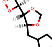
PhEthOH_3854.pdb
