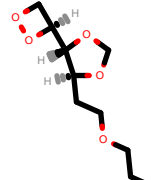
PhEthOH_2590.pdb
