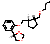
PhEthOH_2890.pdb
