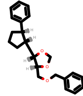
PhEthOH_1190.pdb
