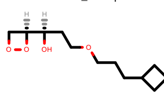
PhEthOH_3642.pdb
