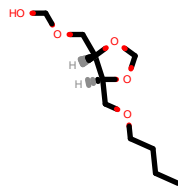
PhEthOH_190.pdb
