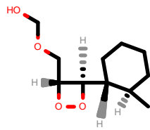
PhEthOH_361.pdb
