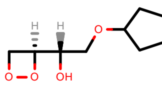
PhEthOH_3894.pdb
