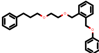
PhEthOH_1054.pdb
