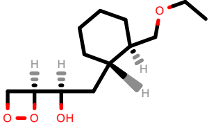
PhEthOH_2508.pdb
