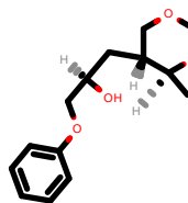
PhEthOH_383.pdb
