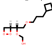
PhEthOH_3643.pdb
