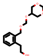
PhEthOH_4721.pdb
