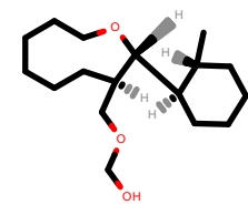
PhEthOH_363.pdb
