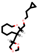
PhEthOH_3189.pdb
