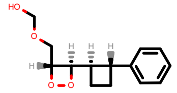
PhEthOH_1159.pdb
