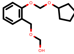
PhEthOH_3886.pdb
