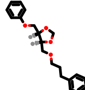
PhEthOH_1054.pdb
