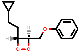
PhEthOH_3069.pdb
