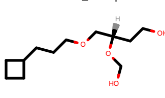
PhEthOH_3630.pdb
