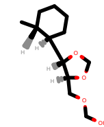
PhEthOH_362.pdb
