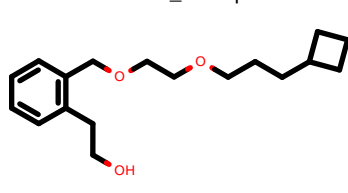
PhEthOH_3629.pdb
