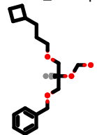
PhEthOH_3624.pdb
