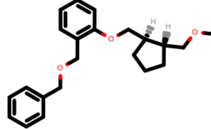
PhEthOH_2026.pdb
