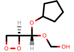
PhEthOH_3895.pdb
