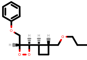
PhEthOH_2821.pdb
