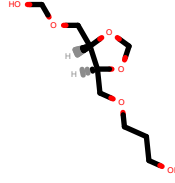
PhEthOH_614.pdb
