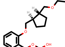
PhEthOH_2454.pdb
