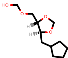
PhEthOH_3848.pdb
