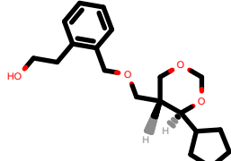
PhEthOH_4213.pdb
