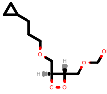
PhEthOH_3217.pdb
