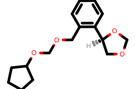
PhEthOH_3899.pdb
