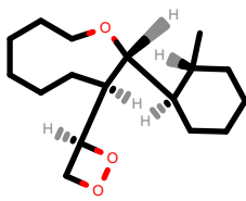
PhEthOH_369.pdb
