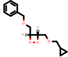
PhEthOH_3121.pdb
