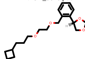
PhEthOH_3647.pdb
