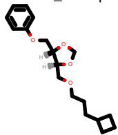
PhEthOH_3620.pdb
