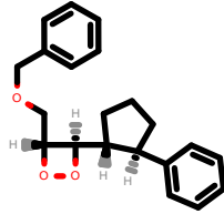
PhEthOH_1189.pdb
