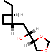
PhEthOH_1590.pdb
