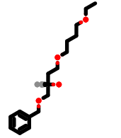
PhEthOH_2321.pdb
