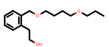
PhEthOH_2659.pdb
