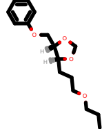
PhEthOH_2654.pdb
