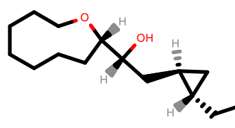
PhEthOH_1554.pdb
