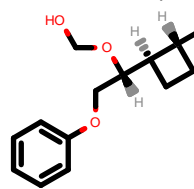
PhEthOH_254.pdb
