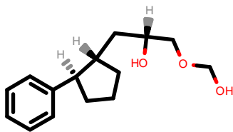
PhEthOH_1200.pdb
