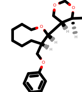
PhEthOH_383.pdb
