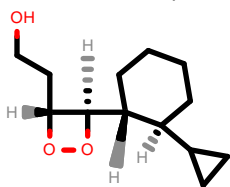
PhEthOH_3333.pdb
