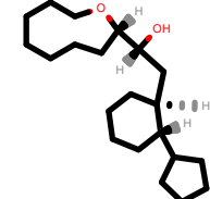
PhEthOH_4200.pdb
