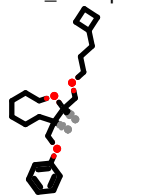
PhEthOH_3621.pdb
