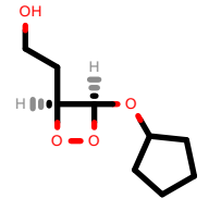
PhEthOH_3883.pdb
