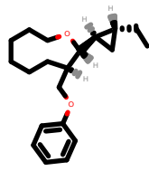
PhEthOH_1521.pdb
