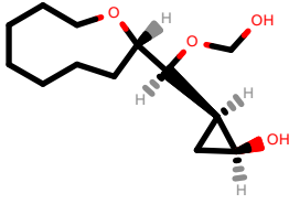
PhEthOH_669.pdb
