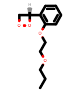
PhEthOH_154.pdb
