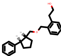
PhEthOH_1189.pdb
