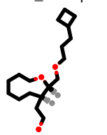
PhEthOH_3633.pdb
