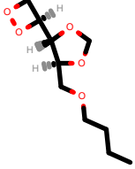
PhEthOH_200.pdb
