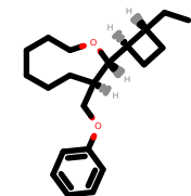
PhEthOH_1559.pdb
