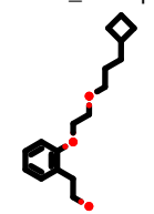
PhEthOH_3628.pdb
