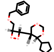
PhEthOH_4213.pdb
