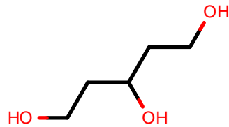
AlkEthOH_c17
