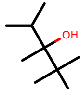
AlkEthOH_c265
