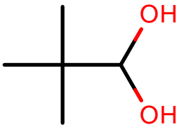
AlkEthOH_c156
