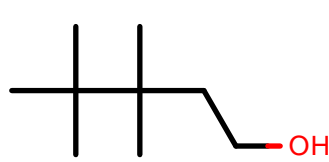
AlkEthOH_c142
