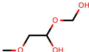
AlkEthOH_c1293
