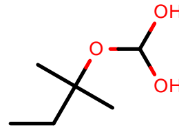
AlkEthOH_c942
