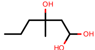
AlkEthOH_c1054
