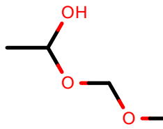
AlkEthOH_c894
