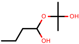
AlkEthOH_c1112
