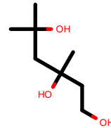
AlkEthOH_c199
