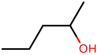
AlkEthOH_c1088
