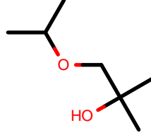
AlkEthOH_c585
