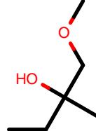
AlkEthOH_c954
