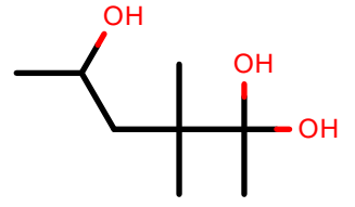
AlkEthOH_c607
