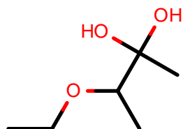
AlkEthOH_c1228
