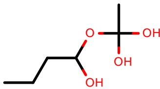
AlkEthOH_c1113
