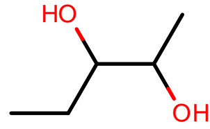
AlkEthOH_c910
