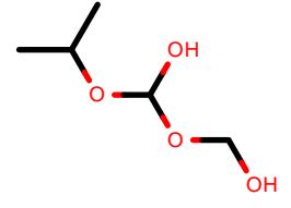
AlkEthOH_c583
