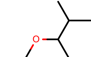
AlkEthOH_c1229
