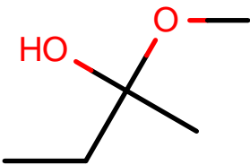
AlkEthOH_c956
