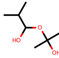
AlkEthOH_c351
