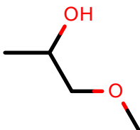
AlkEthOH_c788
