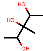
AlkEthOH_c47
