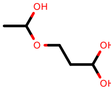
AlkEthOH_c893
