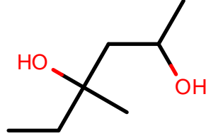
AlkEthOH_c949
