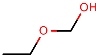
AlkEthOH_c1286
