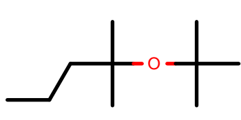
AlkEthOH_c1045
