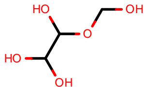
AlkEthOH_c33
