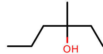
AlkEthOH_c1055
