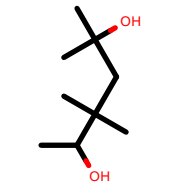
AlkEthOH_c62
