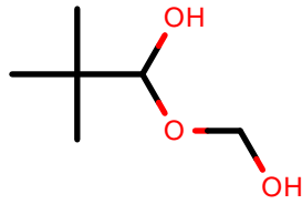
AlkEthOH_c157
