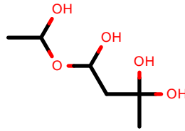
AlkEthOH_c873
