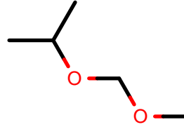
AlkEthOH_c598
