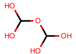
AlkEthOH_c31
