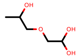
AlkEthOH_c795
