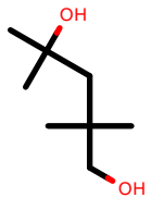
AlkEthOH_c196
