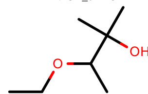
AlkEthOH_c1227
