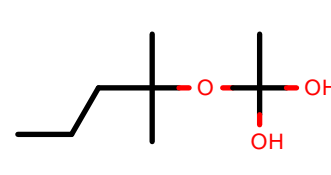
AlkEthOH_c1047
