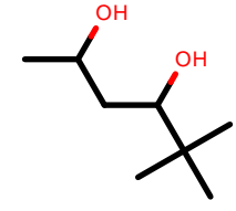
AlkEthOH_c599
