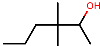
AlkEthOH_c1030
