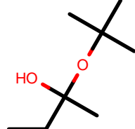
AlkEthOH_c957
