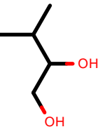
AlkEthOH_c346
