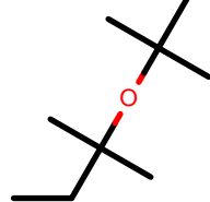
AlkEthOH_c937
