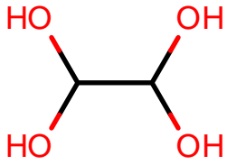
AlkEthOH_c4
