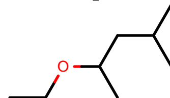
AlkEthOH_c1235
