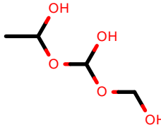
AlkEthOH_c885
