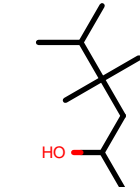
AlkEthOH_c285
