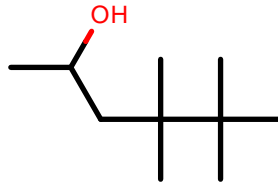
AlkEthOH_c605
