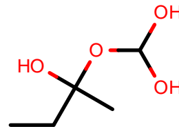
AlkEthOH_c958
