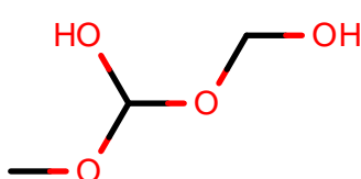
AlkEthOH_c1289
