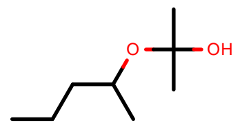
AlkEthOH_c1091
