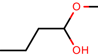
AlkEthOH_c1110
