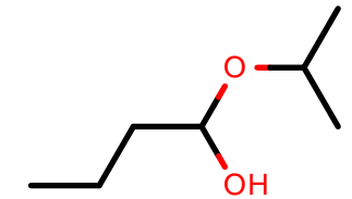
AlkEthOH_c1114
