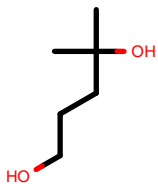
AlkEthOH_c208
