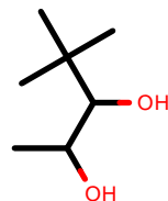
AlkEthOH_c39
