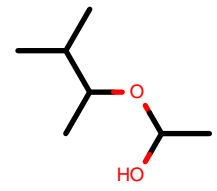
AlkEthOH_c337
