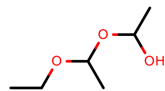
AlkEthOH_c1243
