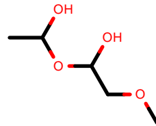
AlkEthOH_c877
