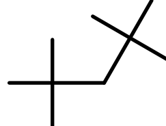
AlkEthOH_c158
