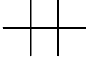
AlkEthOH_c145
