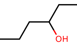
AlkEthOH_c1104
