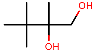
AlkEthOH_c147
