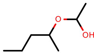
AlkEthOH_c1094
