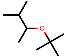
AlkEthOH_c333
