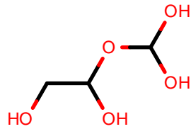
AlkEthOH_c9
