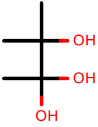
AlkEthOH_c132
