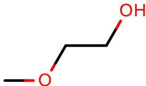
AlkEthOH_c1296
