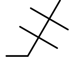
AlkEthOH_c919
