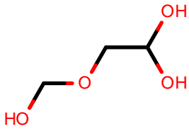
AlkEthOH_c8
