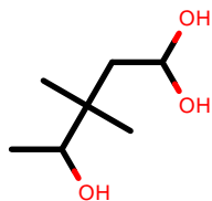
AlkEthOH_c60
