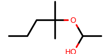
AlkEthOH_c1049
