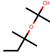
AlkEthOH_c938
