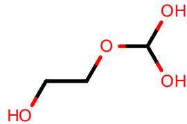
AlkEthOH_c25
