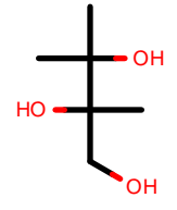
AlkEthOH_c135
