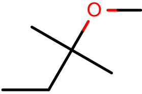
AlkEthOH_c936
