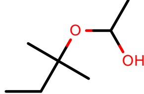
AlkEthOH_c941
