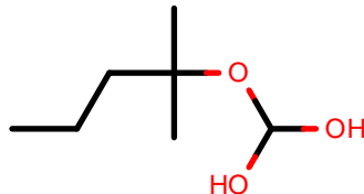
AlkEthOH_c1050
