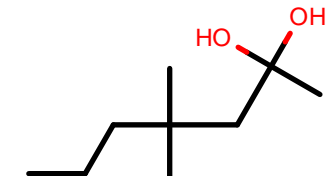
AlkEthOH_c1035
