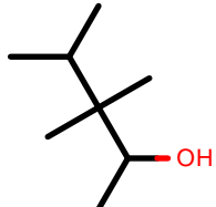
AlkEthOH_c276
