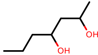
AlkEthOH_c1102
