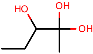
AlkEthOH_c908
