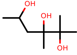
AlkEthOH_c605
