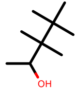
AlkEthOH_c53
