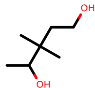
AlkEthOH_c61
