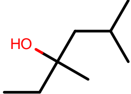
AlkEthOH_c948
