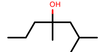
AlkEthOH_c1052
