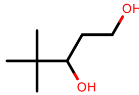
AlkEthOH_c150
