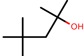
AlkEthOH_c157
