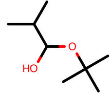
AlkEthOH_c350
