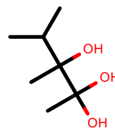
AlkEthOH_c267
