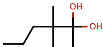
AlkEthOH_c1028
