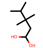
AlkEthOH_c286
