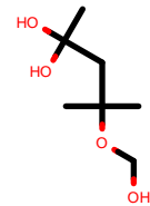
AlkEthOH_c203
