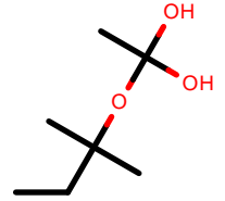
AlkEthOH_c939
