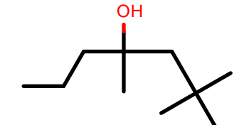
AlkEthOH_c1053
