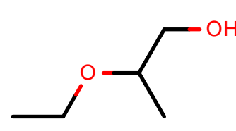
AlkEthOH_c1239
