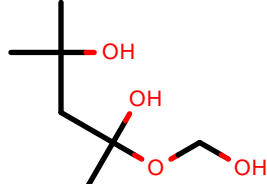
AlkEthOH_c204
