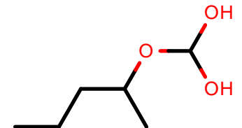
AlkEthOH_c1095
