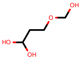
AlkEthOH_c28
