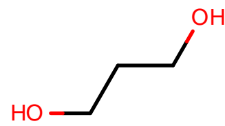
AlkEthOH_c22
