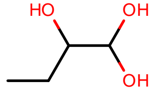
AlkEthOH_c911
