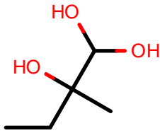
AlkEthOH_c917
