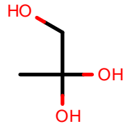
AlkEthOH_c764
