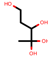
AlkEthOH_c114
