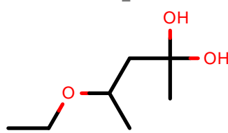
AlkEthOH_c1234
