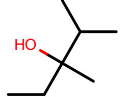
AlkEthOH_c915
