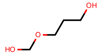
AlkEthOH_c23
