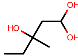
AlkEthOH_c950
