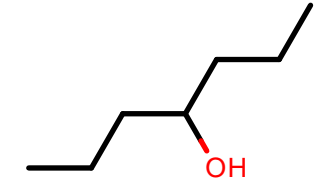
AlkEthOH_c1105
