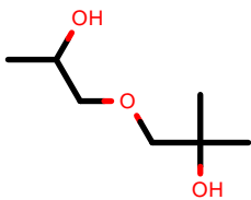
AlkEthOH_c792
