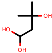
AlkEthOH_c208
