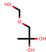
AlkEthOH_c798
