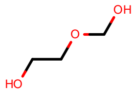
AlkEthOH_c29
