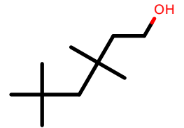
AlkEthOH_c159
