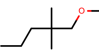
AlkEthOH_c1042
