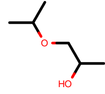
AlkEthOH_c587
