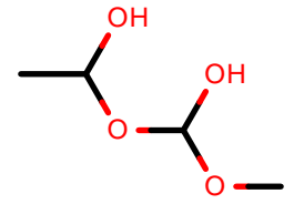
AlkEthOH_c879
