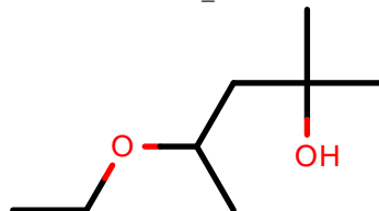
AlkEthOH_c1233
