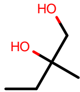
AlkEthOH_c953
