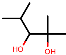
AlkEthOH_c260
