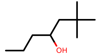
AlkEthOH_c1098
