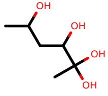
AlkEthOH_c601
