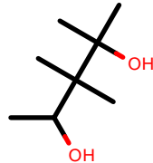
AlkEthOH_c54
