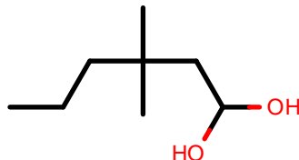
AlkEthOH_c1038
