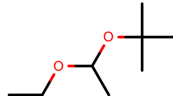
AlkEthOH_c1243
