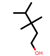
AlkEthOH_c287
