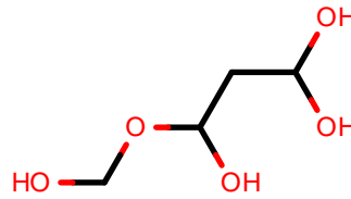
AlkEthOH_c6
