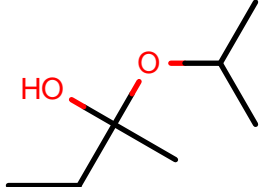
AlkEthOH_c956
