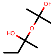
AlkEthOH_c958
