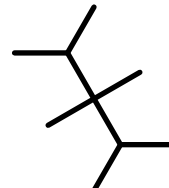
AlkEthOH_c275
