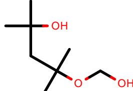
AlkEthOH_c198
