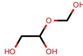
AlkEthOH_c10
