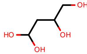
AlkEthOH_c2
