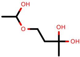
AlkEthOH_c892
