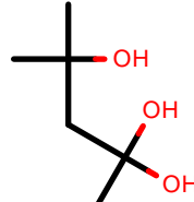
AlkEthOH_c202
