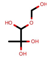
AlkEthOH_c126
