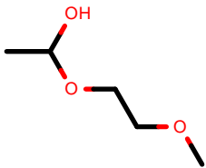
AlkEthOH_c892
