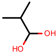
AlkEthOH_c348
