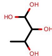
AlkEthOH_c47
