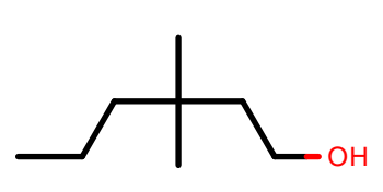
AlkEthOH_c1040
