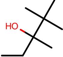
AlkEthOH_c912
