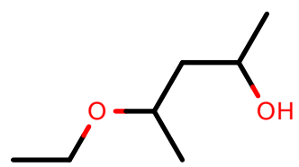
AlkEthOH_c1236
