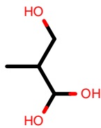
AlkEthOH_c769
