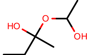
AlkEthOH_c957
