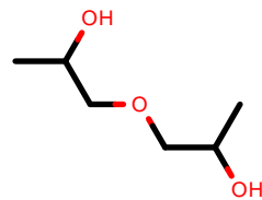
AlkEthOH_c794
