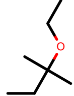
AlkEthOH_c943
