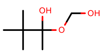
AlkEthOH_c149
