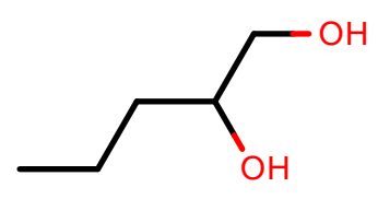
AlkEthOH_c1107
