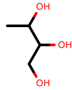
AlkEthOH_c117
