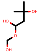
AlkEthOH_c210
