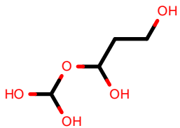
AlkEthOH_c20
