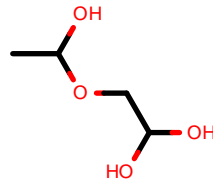
AlkEthOH_c889
