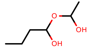
AlkEthOH_c1115
