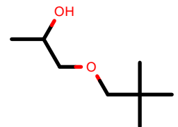
AlkEthOH_c791
