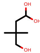
AlkEthOH_c207
