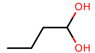
AlkEthOH_c1109
