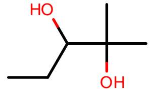
AlkEthOH_c907
