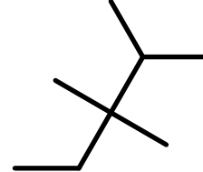
AlkEthOH_c922
