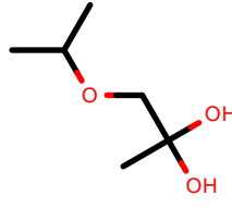
AlkEthOH_c586
