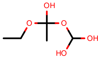
AlkEthOH_c1222
