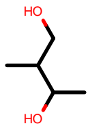
AlkEthOH_c768
