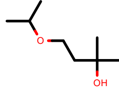
AlkEthOH_c590
