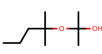
AlkEthOH_c1046
