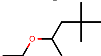
AlkEthOH_c1232
