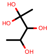
AlkEthOH_c45
