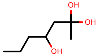
AlkEthOH_c1100
