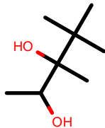
AlkEthOH_c44
