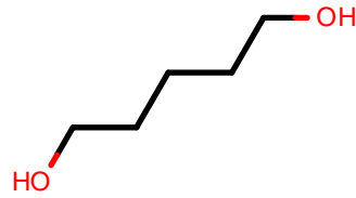
AlkEthOH_c13
