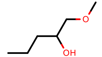
AlkEthOH_c1108
