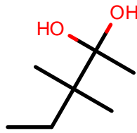
AlkEthOH_c921
