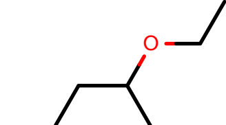
AlkEthOH_c1096
