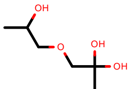
AlkEthOH_c793
