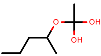
AlkEthOH_c1092
