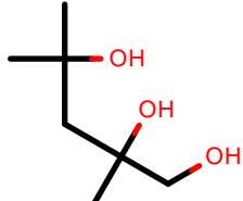
AlkEthOH_c200
