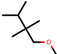
AlkEthOH_c285
