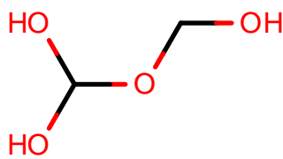
AlkEthOH_c34
