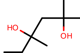
AlkEthOH_c946
