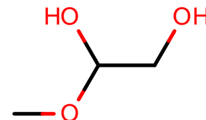
AlkEthOH_c1287
