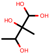
AlkEthOH_c52
