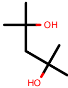
AlkEthOH_c197
