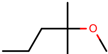
AlkEthOH_c1044
