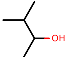
AlkEthOH_c331
