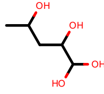
AlkEthOH_c603
