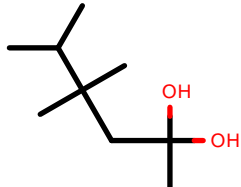
AlkEthOH_c284
