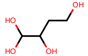
AlkEthOH_c15
