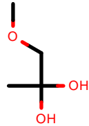
AlkEthOH_c785
