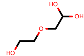
AlkEthOH_c26
