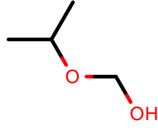
AlkEthOH_c597
