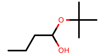
AlkEthOH_c1111
