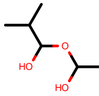
AlkEthOH_c350
