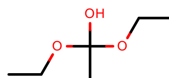
AlkEthOH_c1219
