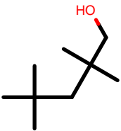
AlkEthOH_c156
