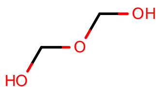
AlkEthOH_c37
