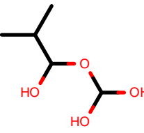
AlkEthOH_c351
