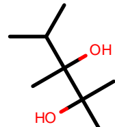
AlkEthOH_c266
