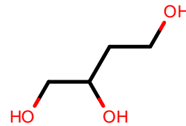
AlkEthOH_c18
