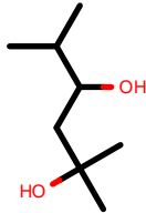
AlkEthOH_c341
