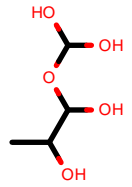
AlkEthOH_c124
