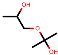
AlkEthOH_c781
