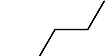
AlkEthOH_c1119
