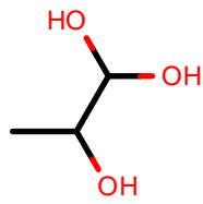
AlkEthOH_c117
