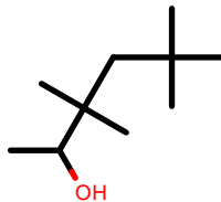
AlkEthOH_c61
