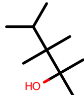
AlkEthOH_c273
