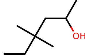
AlkEthOH_c926
