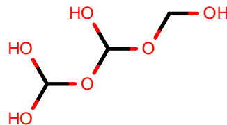
AlkEthOH_c35
