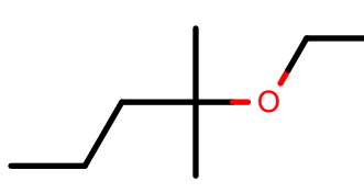
AlkEthOH_c1051
