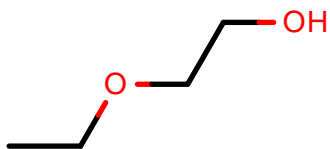
AlkEthOH_c1284
