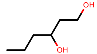
AlkEthOH_c1106
