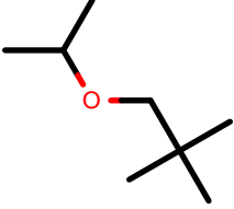
AlkEthOH_c584
