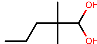
AlkEthOH_c1031
