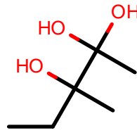
AlkEthOH_c914
