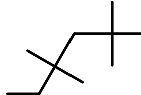
AlkEthOH_c926
