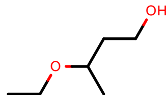
AlkEthOH_c1238
