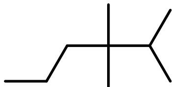
AlkEthOH_c1029
