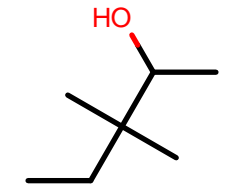
AlkEthOH_c923
