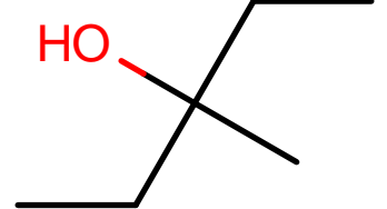
AlkEthOH_c951
