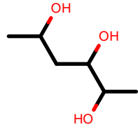
AlkEthOH_c602
