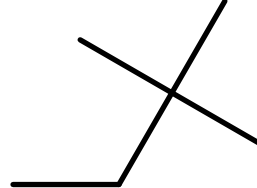
AlkEthOH_c918
