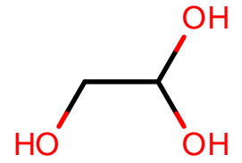
AlkEthOH_c7
