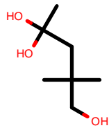
AlkEthOH_c201
