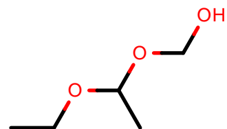
AlkEthOH_c1246
