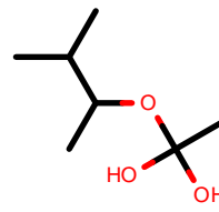
AlkEthOH_c335
