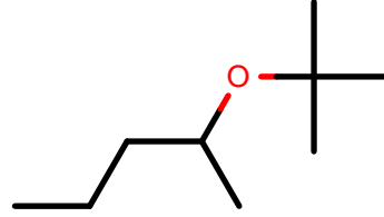
AlkEthOH_c1094
