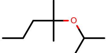
AlkEthOH_c1048
