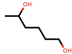
AlkEthOH_c719
