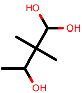
AlkEthOH_c53
