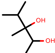
AlkEthOH_c273
