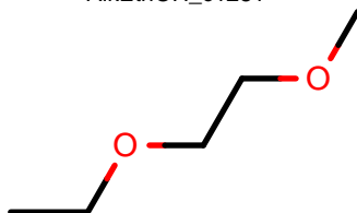
AlkEthOH_c1285
