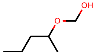
AlkEthOH_c1097
