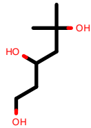
AlkEthOH_c205
