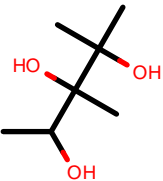
AlkEthOH_c45
