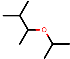
AlkEthOH_c336
