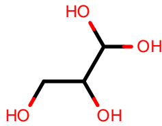
AlkEthOH_c1
