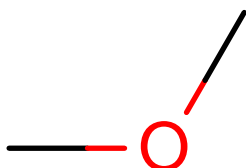
AlkEthOH_c1285
