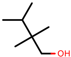
AlkEthOH_c284
