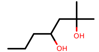
AlkEthOH_c1099
