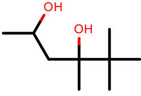
AlkEthOH_c604
