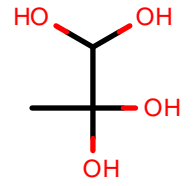
AlkEthOH_c119
