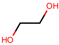
AlkEthOH_c24
