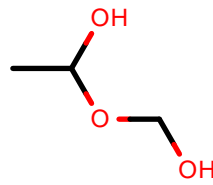
AlkEthOH_c893
