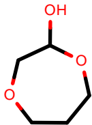
AlkEthOH_r144
