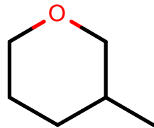
AlkEthOH_r965
