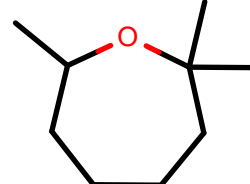
AlkEthOH_r871
