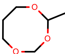
AlkEthOH_r1140
