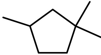
AlkEthOH_r841
