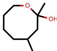
AlkEthOH_r926
