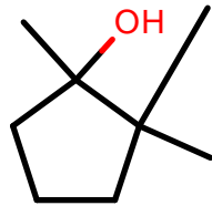
AlkEthOH_r325
