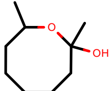
AlkEthOH_r885
