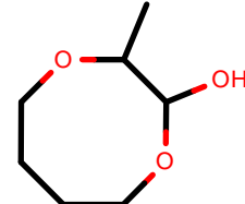
AlkEthOH_r766
