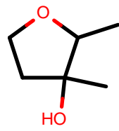
AlkEthOH_r753
