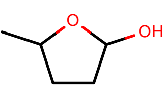
AlkEthOH_r848
