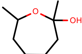
AlkEthOH_r872
