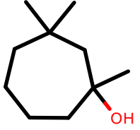
AlkEthOH_r332
