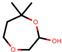
AlkEthOH_r536
