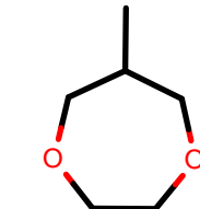
AlkEthOH_r1103
