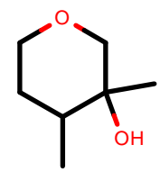
AlkEthOH_r1018
