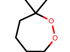
AlkEthOH_r459
