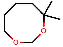
AlkEthOH_r455
