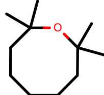
AlkEthOH_r349
