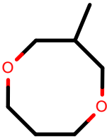
AlkEthOH_r1092
