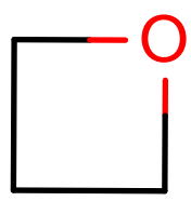
AlkEthOH_r131
