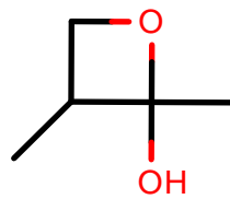
AlkEthOH_r1062
