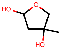
AlkEthOH_r265
