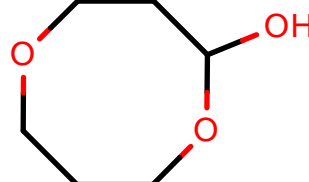
AlkEthOH_r146
