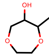
AlkEthOH_r766
