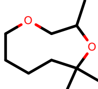
AlkEthOH_r1077
