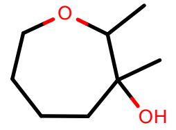
AlkEthOH_r747
