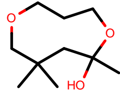
AlkEthOH_r276
