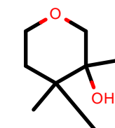
AlkEthOH_r539
