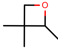
AlkEthOH_r758
