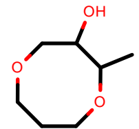
AlkEthOH_r763
