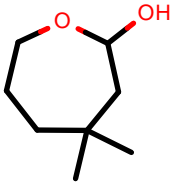
AlkEthOH_r468
