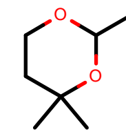
AlkEthOH_r1119
