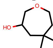
AlkEthOH_r531
