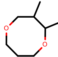
AlkEthOH_r1095
