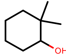
AlkEthOH_r346
