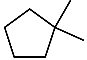
AlkEthOH_r327
