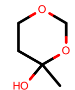
AlkEthOH_r571
