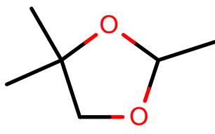
AlkEthOH_r1116
