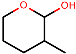
AlkEthOH_r973
