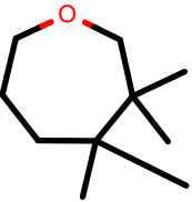
AlkEthOH_r492
