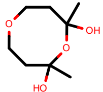
AlkEthOH_r556
