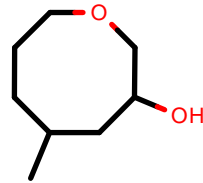
AlkEthOH_r977
