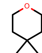
AlkEthOH_r541
