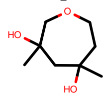
AlkEthOH_r530
