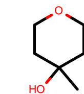
AlkEthOH_r542
