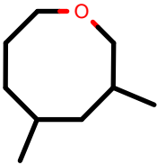
AlkEthOH_r976
