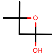
AlkEthOH_r257
