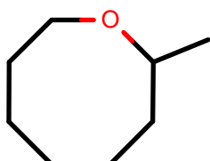
AlkEthOH_r904
