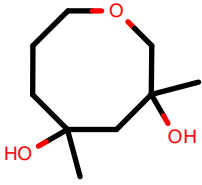
AlkEthOH_r484
