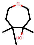
AlkEthOH_r556
