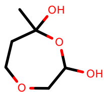
AlkEthOH_r537
