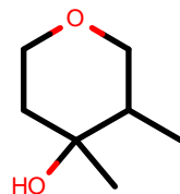
AlkEthOH_r1069
