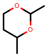
AlkEthOH_r1001
