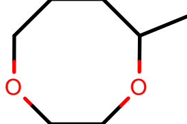
AlkEthOH_r989
