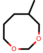
AlkEthOH_r991
