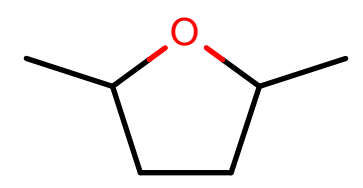
AlkEthOH_r847
