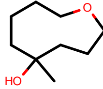
AlkEthOH_r454
