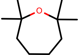
AlkEthOH_r336
