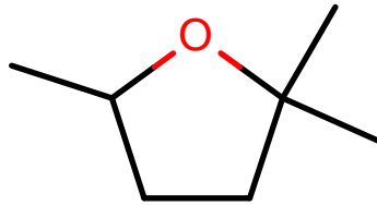
AlkEthOH_r845
