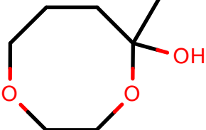
AlkEthOH_r504
