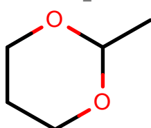
AlkEthOH_r1136
