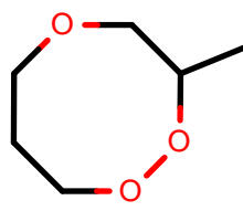
AlkEthOH_r1097
