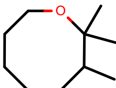
AlkEthOH_r917
