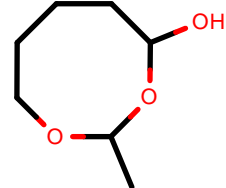
AlkEthOH_r1127
