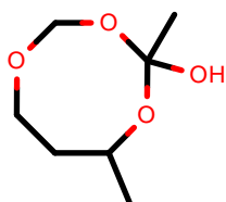
AlkEthOH_r1040
