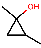
AlkEthOH_r838
