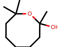
AlkEthOH_r350
