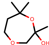
AlkEthOH_r534
