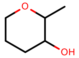
AlkEthOH_r751
