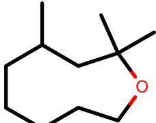
AlkEthOH_r908
