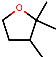
AlkEthOH_r1004
