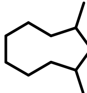
AlkEthOH_r895
