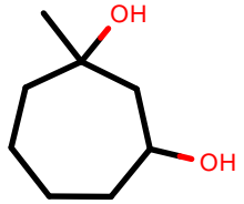
AlkEthOH_r335
