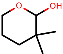
AlkEthOH_r476
