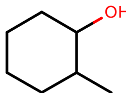
AlkEthOH_r875
