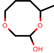
AlkEthOH_r981
