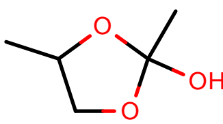
AlkEthOH_r1053
