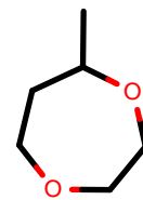
AlkEthOH_r1031
