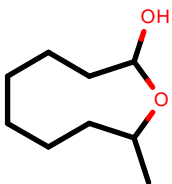
AlkEthOH_r900
