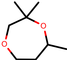
AlkEthOH_r1012
