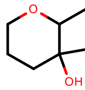
AlkEthOH_r750
