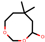
AlkEthOH_r575
