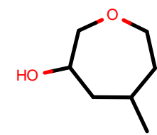
AlkEthOH_r1011
