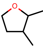
AlkEthOH_r1006
