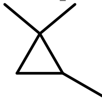
AlkEthOH_r837
