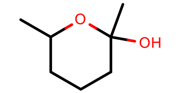
AlkEthOH_r859
