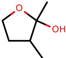
AlkEthOH_r1005
