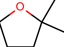
AlkEthOH_r463
