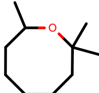
AlkEthOH_r884
