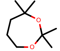
AlkEthOH_r470
