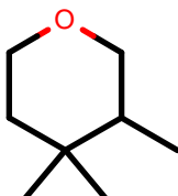
AlkEthOH_r1068
