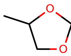
AlkEthOH_r1110
