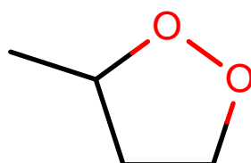
AlkEthOH_r1049
