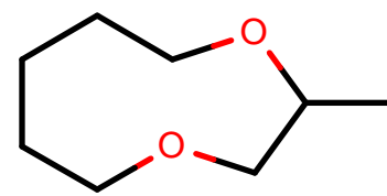
AlkEthOH_r1079
