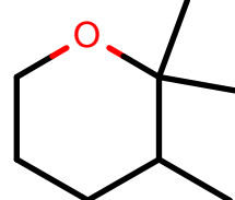
AlkEthOH_r966
