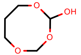
AlkEthOH_r159
