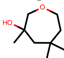
AlkEthOH_r529
