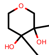
AlkEthOH_r540
