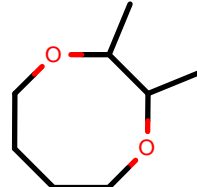
AlkEthOH_r765
