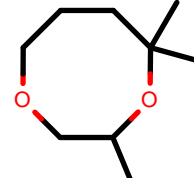
AlkEthOH_r1071
