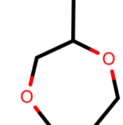
AlkEthOH_r1087
