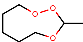
AlkEthOH_r1129
