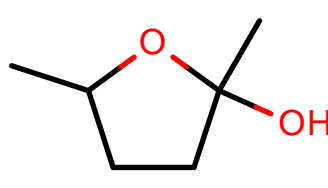
AlkEthOH_r846
