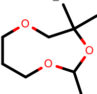
AlkEthOH_r1137
