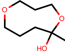
AlkEthOH_r502
