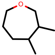
AlkEthOH_r985
