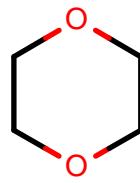
AlkEthOH_r150
