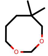
AlkEthOH_r507
