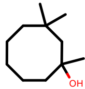
AlkEthOH_r349
