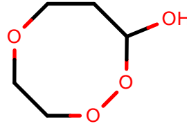
AlkEthOH_r158
