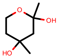
AlkEthOH_r513
