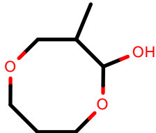
AlkEthOH_r1096
