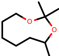
AlkEthOH_r912
