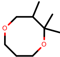
AlkEthOH_r1093
