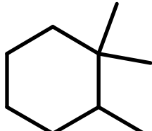
AlkEthOH_r872
