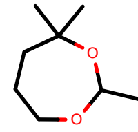
AlkEthOH_r1118
