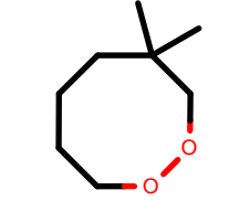
AlkEthOH_r461
