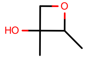
AlkEthOH_r759
