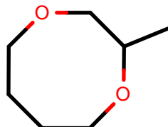
AlkEthOH_r1084
