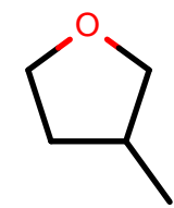
AlkEthOH_r1003
