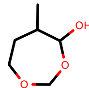
AlkEthOH_r1047
