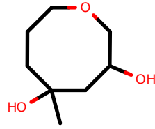
AlkEthOH_r486
