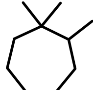
AlkEthOH_r885
