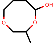
AlkEthOH_r1073
