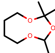
AlkEthOH_r1131
