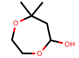
AlkEthOH_r279
