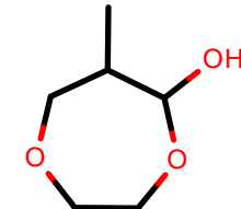
AlkEthOH_r1107
