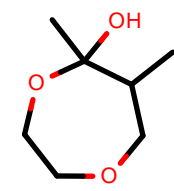
AlkEthOH_r1105
