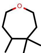
AlkEthOH_r1025
