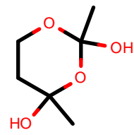
AlkEthOH_r522
