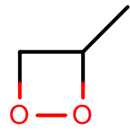
AlkEthOH_r1113
