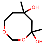
AlkEthOH_r574
