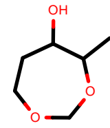
AlkEthOH_r757
