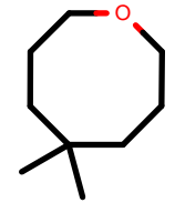
AlkEthOH_r499
