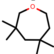
AlkEthOH_r528
