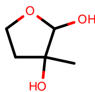
AlkEthOH_r527
