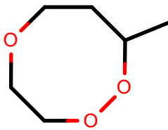
AlkEthOH_r1033
