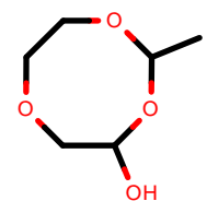
AlkEthOH_r1149
