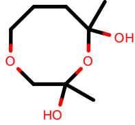
AlkEthOH_r489
