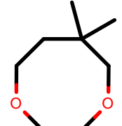
AlkEthOH_r566
