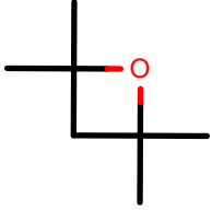
AlkEthOH_r260
