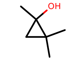
AlkEthOH_r287
