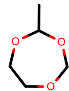
AlkEthOH_r1150
