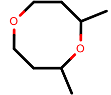
AlkEthOH_r1023
