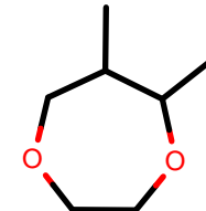
AlkEthOH_r1106
