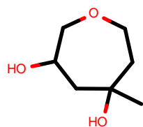
AlkEthOH_r532
