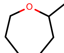
AlkEthOH_r907
