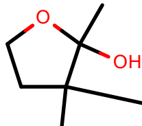
AlkEthOH_r522
