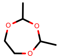
AlkEthOH_r1145
