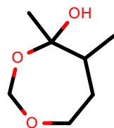
AlkEthOH_r1045
