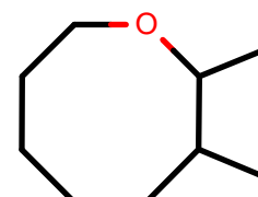
AlkEthOH_r919
