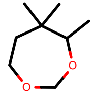
AlkEthOH_r755
