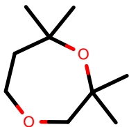
AlkEthOH_r533
