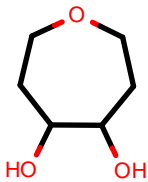
AlkEthOH_r144
