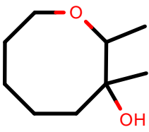
AlkEthOH_r744
