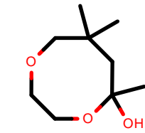
AlkEthOH_r286
