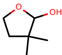
AlkEthOH_r526
