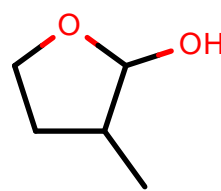
AlkEthOH_r1007
