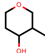
AlkEthOH_r1070
