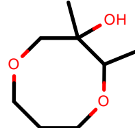
AlkEthOH_r762
