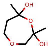
AlkEthOH_r535
