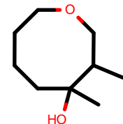
AlkEthOH_r1077
