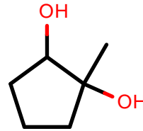
AlkEthOH_r326
