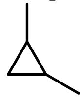
AlkEthOH_r839
