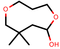
AlkEthOH_r278
