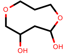
AlkEthOH_r139
