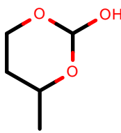
AlkEthOH_r1002
