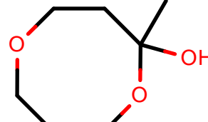
AlkEthOH_r563
