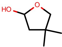
AlkEthOH_r264
