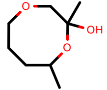
AlkEthOH_r979
