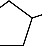
AlkEthOH_r862
