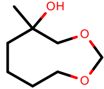
AlkEthOH_r458
