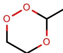
AlkEthOH_r1151
