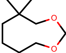
AlkEthOH_r457
