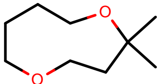
AlkEthOH_r560
