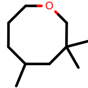
AlkEthOH_r974
