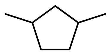
AlkEthOH_r843
