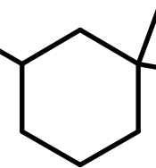
AlkEthOH_r854
