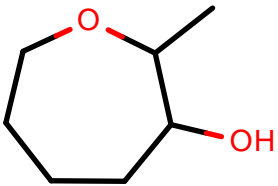
AlkEthOH_r748
