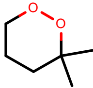
AlkEthOH_r509
