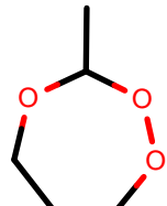
AlkEthOH_r1141
