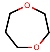
AlkEthOH_r151
