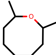
AlkEthOH_r886
