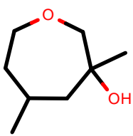
AlkEthOH_r1009
