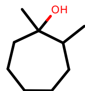
AlkEthOH_r886
