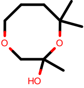
AlkEthOH_r488
