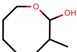
AlkEthOH_r920
