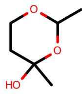
AlkEthOH_r1116
