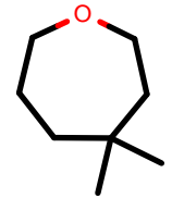
AlkEthOH_r495
