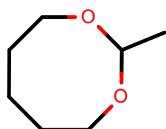
AlkEthOH_r1128
