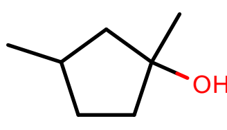
AlkEthOH_r842
