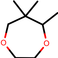
AlkEthOH_r764
