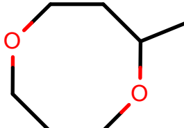
AlkEthOH_r1030
