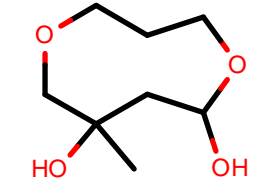
AlkEthOH_r279
