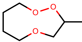
AlkEthOH_r1086
