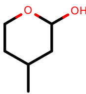
AlkEthOH_r998
