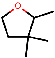
AlkEthOH_r752
