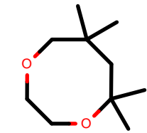
AlkEthOH_r285
