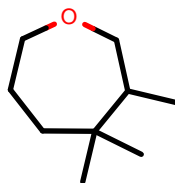
AlkEthOH_r1074
