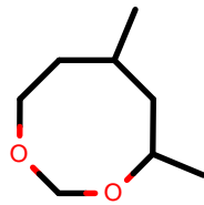
AlkEthOH_r1041
