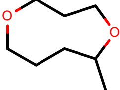
AlkEthOH_r988
