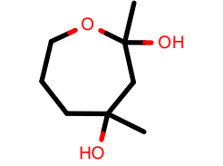
AlkEthOH_r467
