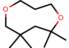
AlkEthOH_r275
