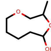
AlkEthOH_r1079
