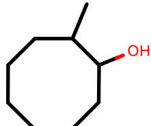
AlkEthOH_r901
