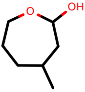
AlkEthOH_r964
