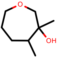
AlkEthOH_r984
