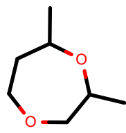
AlkEthOH_r1014
