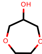
AlkEthOH_r137
