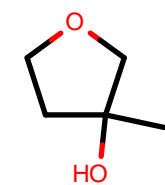
AlkEthOH_r525
