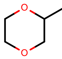
AlkEthOH_r1098
