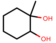
AlkEthOH_r347
