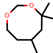
AlkEthOH_r1035
