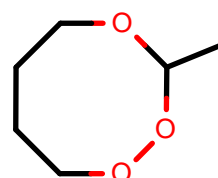
AlkEthOH_r1135
