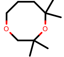
AlkEthOH_r487
