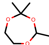
AlkEthOH_r1143
