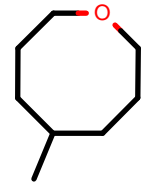
AlkEthOH_r987
