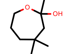
AlkEthOH_r466
