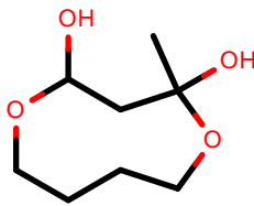
AlkEthOH_r274
