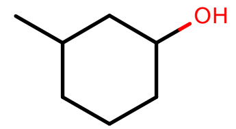
AlkEthOH_r857
