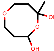
AlkEthOH_r558
