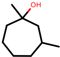
AlkEthOH_r868
