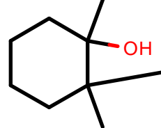
AlkEthOH_r342
