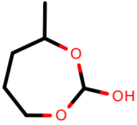
AlkEthOH_r964
