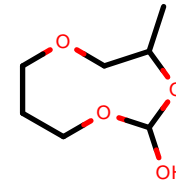
AlkEthOH_r1087
