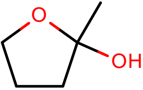
AlkEthOH_r464
