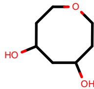
AlkEthOH_r145
