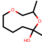
AlkEthOH_r1078
