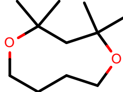
AlkEthOH_r266
