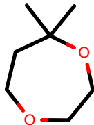
AlkEthOH_r564
