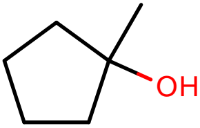
AlkEthOH_r324
