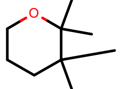
AlkEthOH_r475
