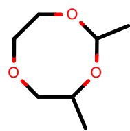
AlkEthOH_r1101
