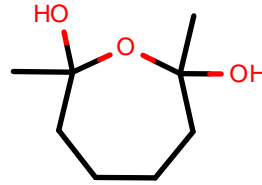
AlkEthOH_r338
