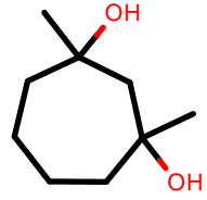
AlkEthOH_r333
