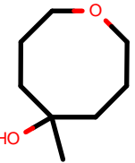
AlkEthOH_r500
