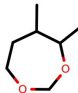
AlkEthOH_r1046
