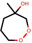
AlkEthOH_r508
