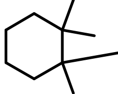
AlkEthOH_r341
