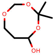
AlkEthOH_r737
