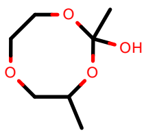
AlkEthOH_r1100
