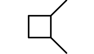
AlkEthOH_r852
