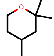
AlkEthOH_r991
