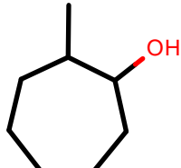
AlkEthOH_r892
