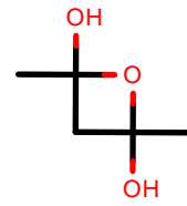
AlkEthOH_r258
