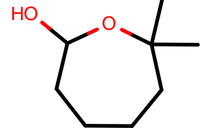
AlkEthOH_r339
