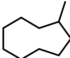
AlkEthOH_r902
