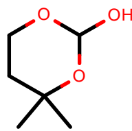
AlkEthOH_r523
