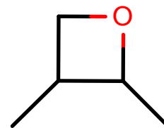
AlkEthOH_r1063
