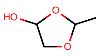
AlkEthOH_r1118
