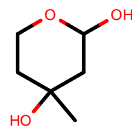
AlkEthOH_r515
