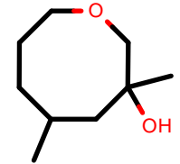
AlkEthOH_r975
