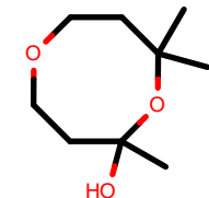
AlkEthOH_r551
