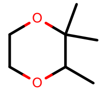
AlkEthOH_r767
