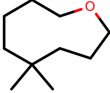
AlkEthOH_r453
