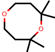
AlkEthOH_r550
