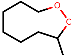
AlkEthOH_r906
