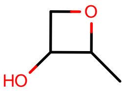
AlkEthOH_r760
