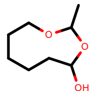
AlkEthOH_r1126
