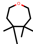
AlkEthOH_r559
