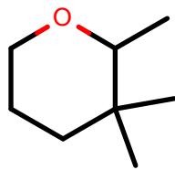
AlkEthOH_r749
