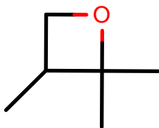
AlkEthOH_r1061
