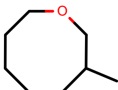
AlkEthOH_r916
