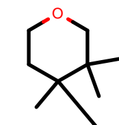
AlkEthOH_r538
