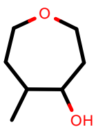
AlkEthOH_r1028
