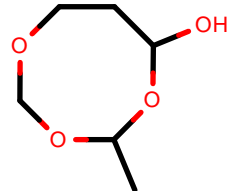
AlkEthOH_r1155
