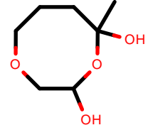
AlkEthOH_r491
