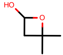
AlkEthOH_r259
