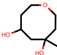
AlkEthOH_r549
