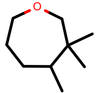
AlkEthOH_r983
