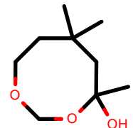
AlkEthOH_r573
