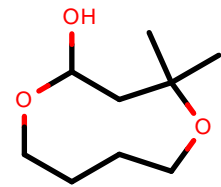
AlkEthOH_r273
