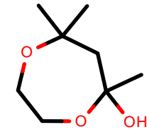
AlkEthOH_r277
