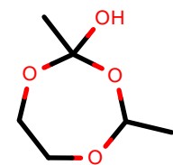
AlkEthOH_r1144
