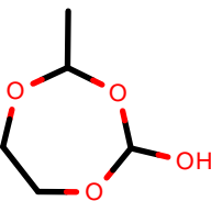
AlkEthOH_r1146
