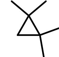
AlkEthOH_r286
