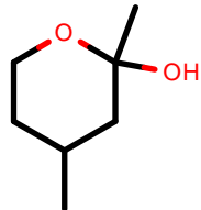
AlkEthOH_r996
