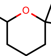
AlkEthOH_r858
