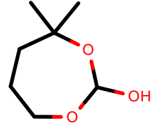
AlkEthOH_r473
