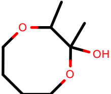
AlkEthOH_r764
