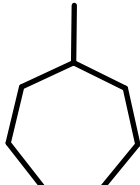
AlkEthOH_r884
