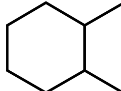
AlkEthOH_r874
