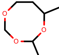
AlkEthOH_r1041
