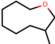
AlkEthOH_r905
