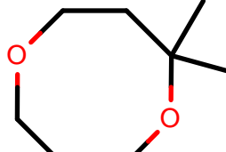
AlkEthOH_r562
