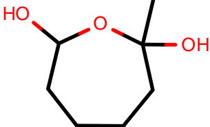
AlkEthOH_r340
