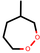
AlkEthOH_r989
