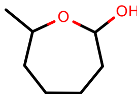
AlkEthOH_r874
