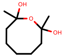
AlkEthOH_r351
