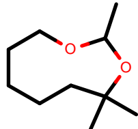
AlkEthOH_r1128
