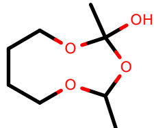
AlkEthOH_r1136
