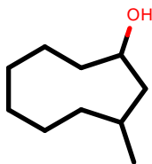
AlkEthOH_r892
