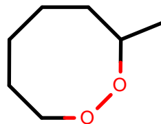
AlkEthOH_r922
