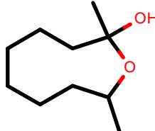
AlkEthOH_r894
