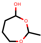
AlkEthOH_r1120
