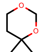
AlkEthOH_r570
