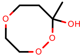
AlkEthOH_r569
