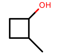
AlkEthOH_r853
