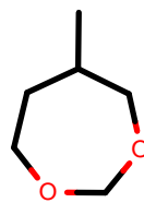
AlkEthOH_r1043
