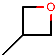
AlkEthOH_r1060
