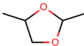
AlkEthOH_r1054
