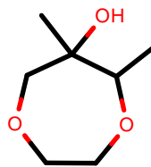
AlkEthOH_r765
