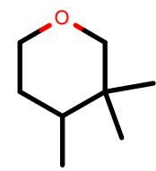
AlkEthOH_r1017
