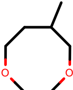
AlkEthOH_r1032
