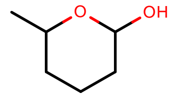
AlkEthOH_r861
