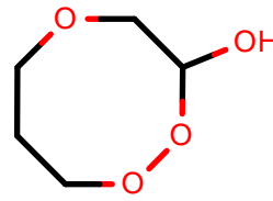
AlkEthOH_r146
