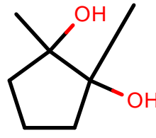
AlkEthOH_r326
