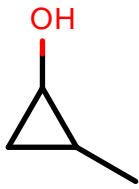
AlkEthOH_r840
