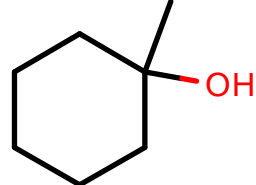
AlkEthOH_r345
