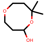
AlkEthOH_r557
