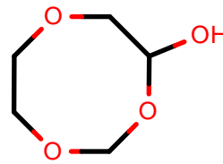
AlkEthOH_r158
