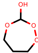
AlkEthOH_r130
