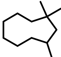
AlkEthOH_r893
