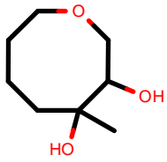
AlkEthOH_r452
