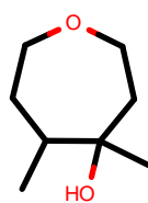
AlkEthOH_r1026
