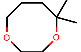
AlkEthOH_r503
