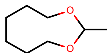
AlkEthOH_r1127
