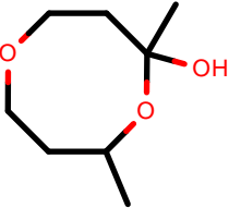
AlkEthOH_r1022
