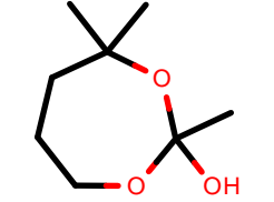
AlkEthOH_r471
