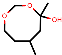
AlkEthOH_r1040
