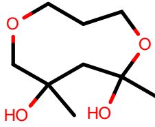
AlkEthOH_r277
