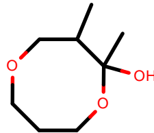
AlkEthOH_r1094
