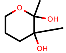
AlkEthOH_r477
