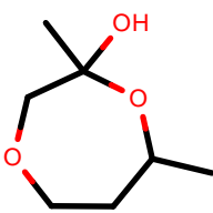
AlkEthOH_r1013
