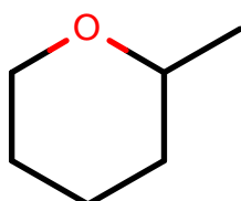
AlkEthOH_r924
