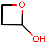
AlkEthOH_r136
