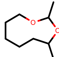
AlkEthOH_r914
