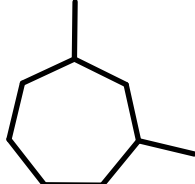
AlkEthOH_r869
