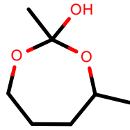
AlkEthOH_r966
