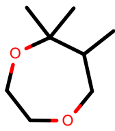
AlkEthOH_r1104
