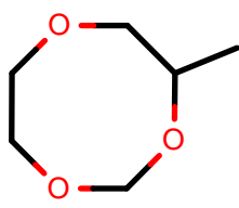
AlkEthOH_r1108
