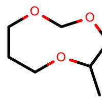
AlkEthOH_r1111
