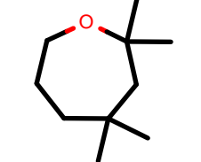
AlkEthOH_r465
