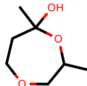
AlkEthOH_r1062
