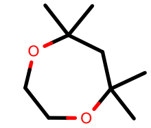
AlkEthOH_r276
