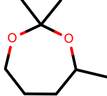
AlkEthOH_r965
