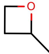
AlkEthOH_r990
