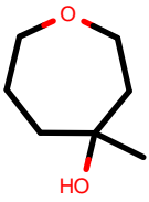
AlkEthOH_r496
