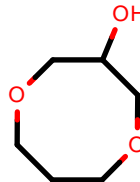
AlkEthOH_r138
