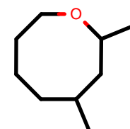
AlkEthOH_r927
