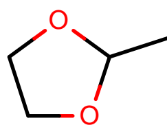
AlkEthOH_r1142
