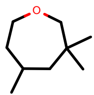
AlkEthOH_r1008
