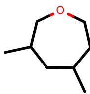
AlkEthOH_r1010
