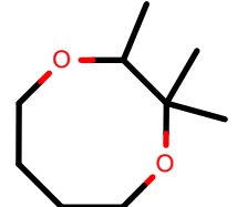
AlkEthOH_r767
