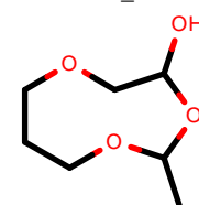
AlkEthOH_r1139
