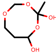
AlkEthOH_r738
