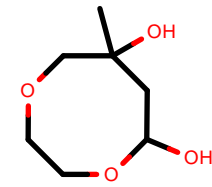
AlkEthOH_r285
