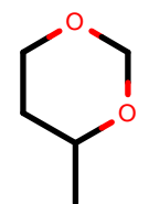
AlkEthOH_r1034
