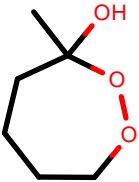
AlkEthOH_r460
