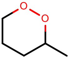
AlkEthOH_r988
