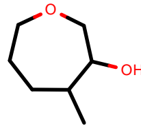
AlkEthOH_r986
