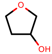
AlkEthOH_r147
