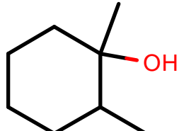
AlkEthOH_r873
