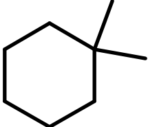
AlkEthOH_r344
