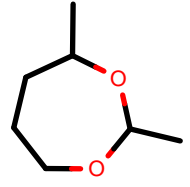
AlkEthOH_r967
