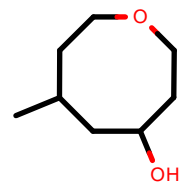
AlkEthOH_r1020
