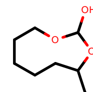
AlkEthOH_r915
