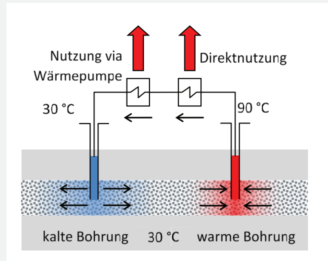
Abb. 4: Prinzip der saisonalen Wärmespeicherung in Aquiferen (Temperaturangaben sind beispielhaft): links – Einspeicherung, rechts – Ausspeicherung
