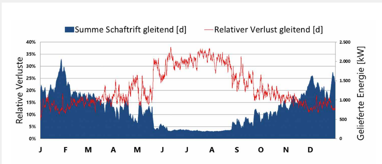
Abb. 2: Wärmelieferung und relative Netzwärmlverluste im Jahresgang
