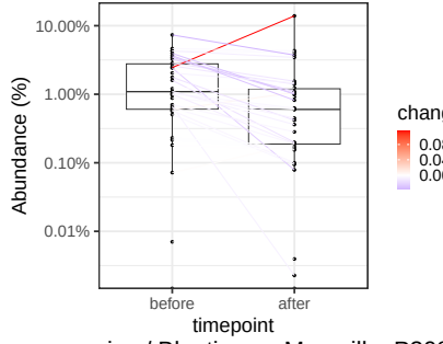
rice / Blautia_sp_Marseille_P3087
