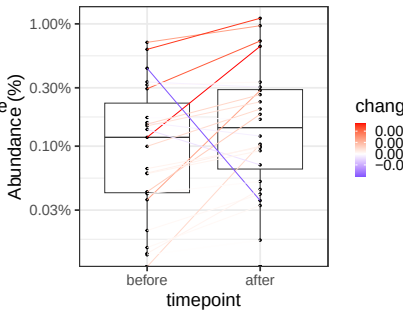
oat / Blautia_massiliensis
