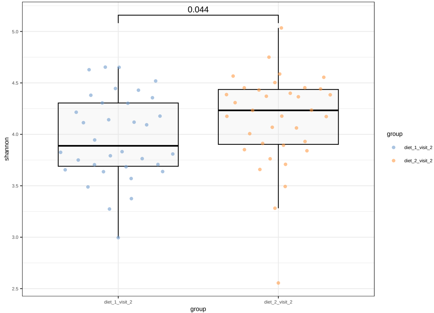
shannon Diversity: diet_1_visit_2 vs diet_2_visit_2
