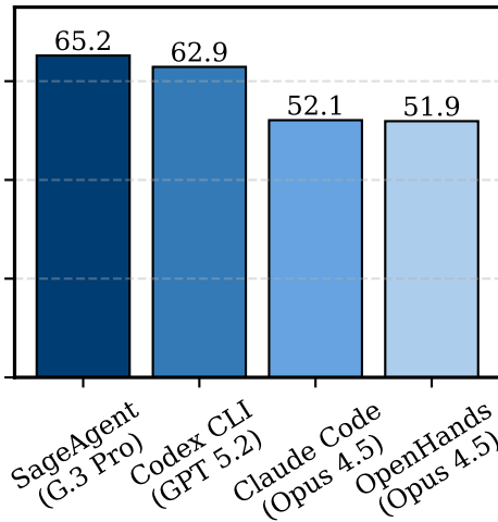
Terminal-Bench 2.0
