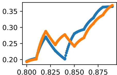
forcesetglut_med3_rfiber_length
