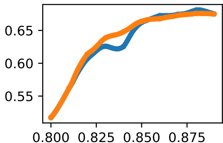
forcesetglut_med2_ractivation
