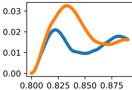
jointsetmtp_rmtmp_angle_rspeed
