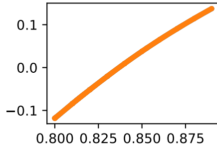
jointsethip_lhip_adduction_lspeed
