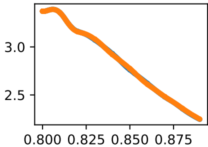
jointsethip_lhip_flexion_lspeed
