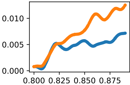
jointsethip_lhip_flexion_lspeed
