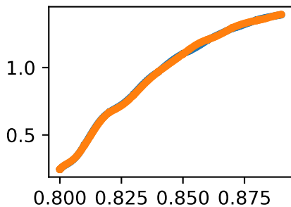
jointsetsubtalar_rsubtalar_angle_rvalue
