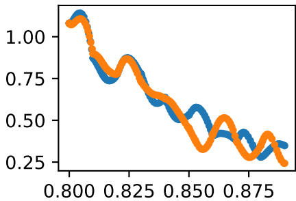
jointsetmtp_rmtmp_angle_rvalue
