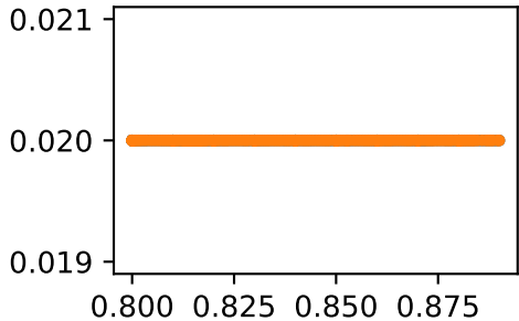
forcesetsar_rfiber_length
