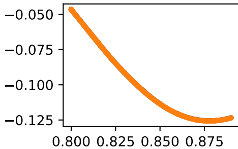
jointsethip_lhip_adduction_lvalue
