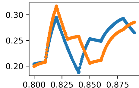
forcesetbifemlh_rfiber_length
