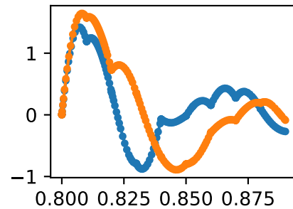
jointsethip_lhip_flexion_lvalue
