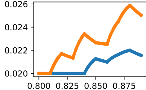
forcesetadd_mag2_rfiber_length
