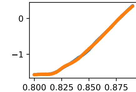
jointsethip_lhip_adduction_lspeed
