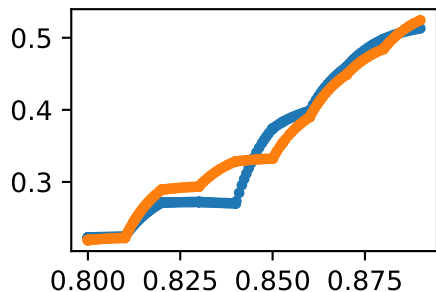
forcesetglut_med2_rfiber_length
