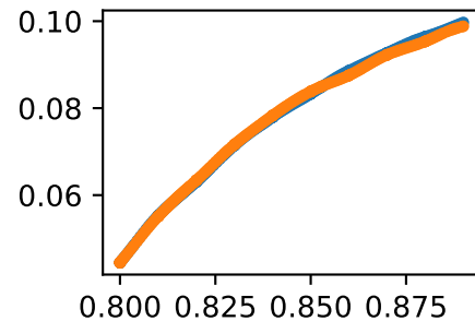
jointsetsubtalar_rsubtalar_angle_rspeed
