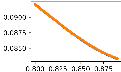
forcesetadd_mag2_rfiber_length
