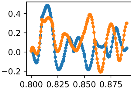
jointsethip_lhip_adduction_lvalue
