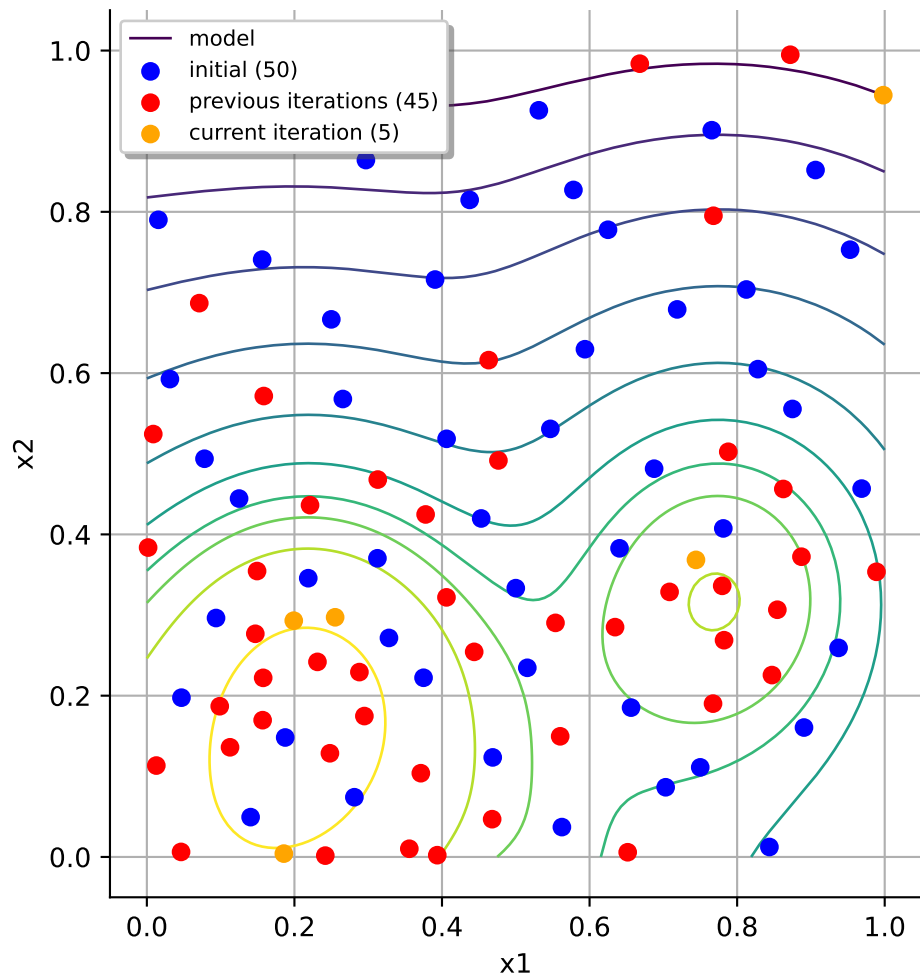
LOLA-Voronoi iteration #10 N=100
