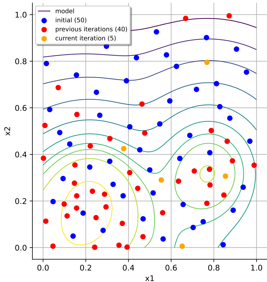
LOLA-Voronoi iteration #9 N=95
