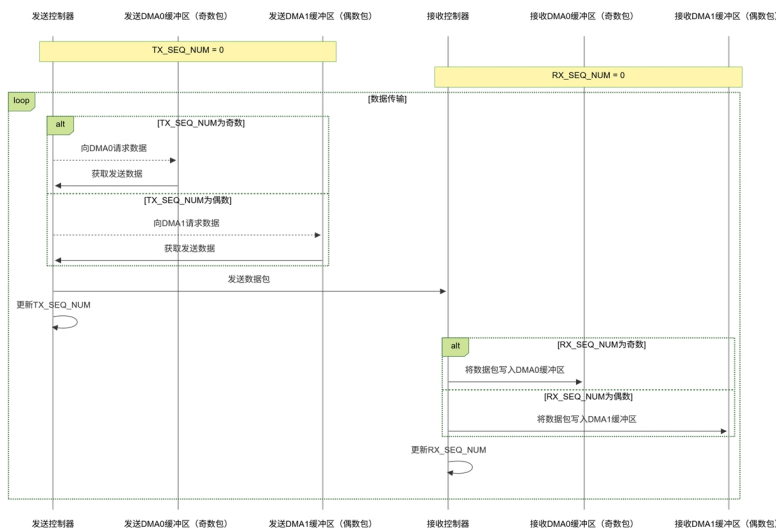
图 1-1 双缓冲传输时序图 Chnn
