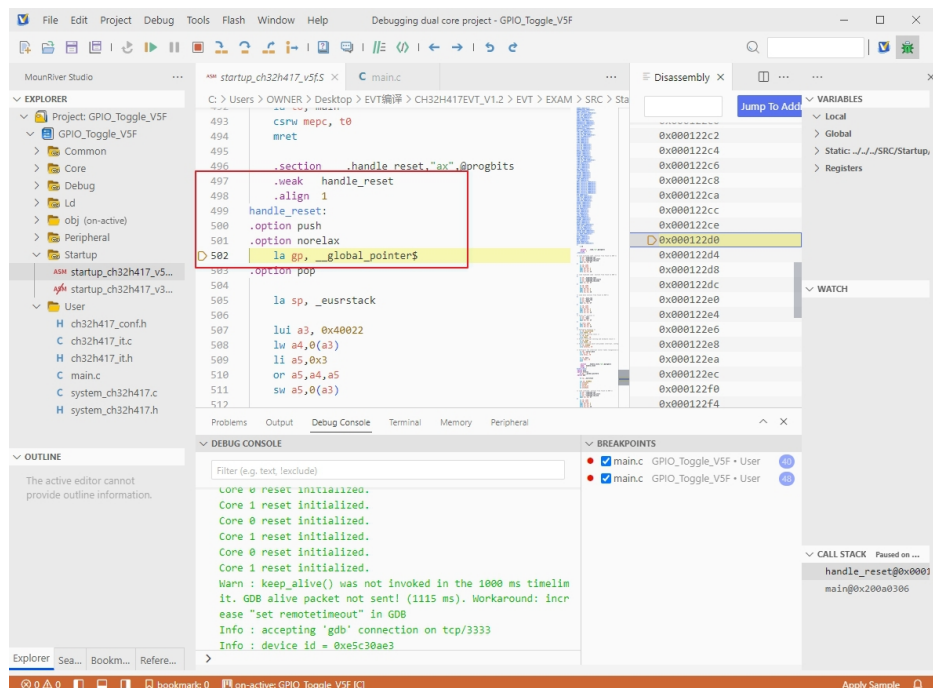
图 2-4 V5 核默认临时断点示意图
