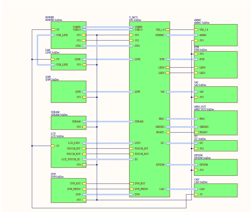
图 2-1 硬件框图
