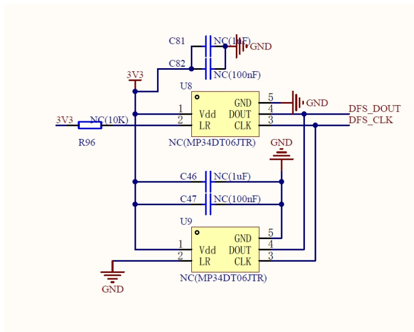
图 2-10 DFSDM 接口麦克风示意图
