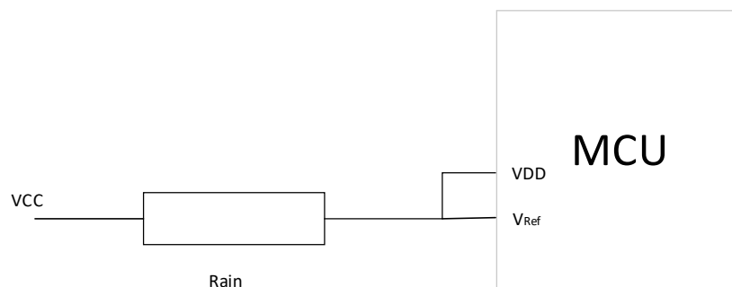
图错误!文档中没有指定样式的文字。-7 供电拓扑结构
