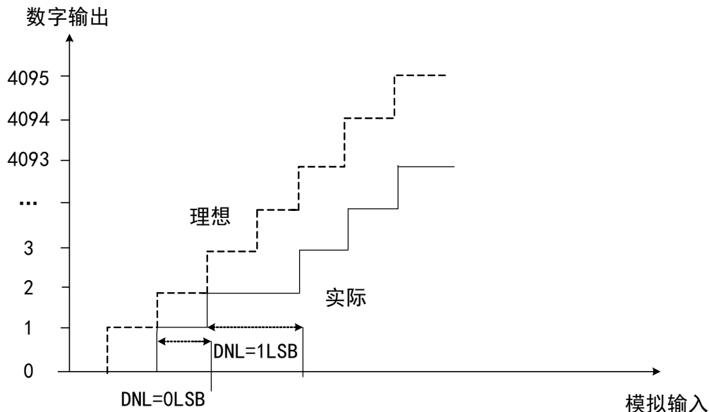
图 1-4 ADC 微分误差
