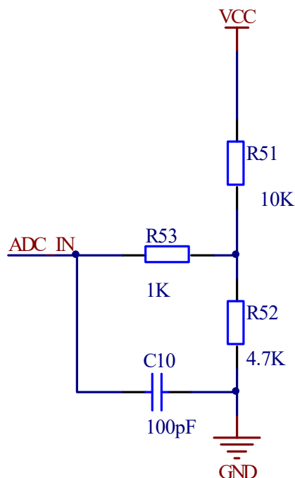
图错误!文档中没有指定样式的文字。 -8 ADC 采样电路
