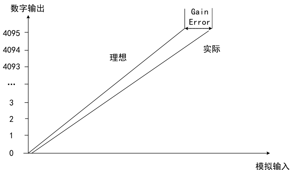
图 1-3 ADC 增益误差
