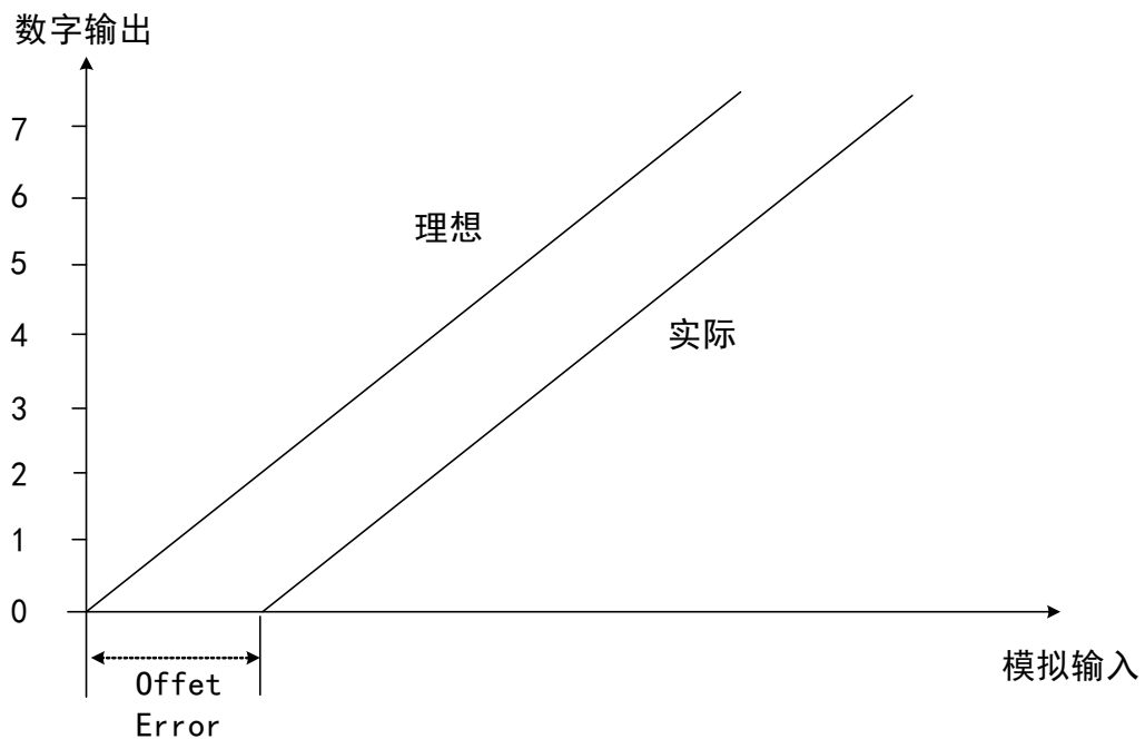
图 1-2 ADC 失调误差
