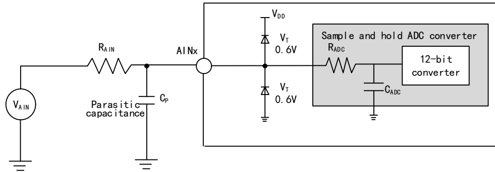
图错误!文档中没有指定样式的文字。-9 ADC 拓扑结构
