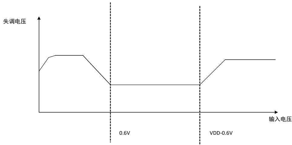
图错误!文档中没有指定样式的文字。-11 跟随器输入电压与失调电压
