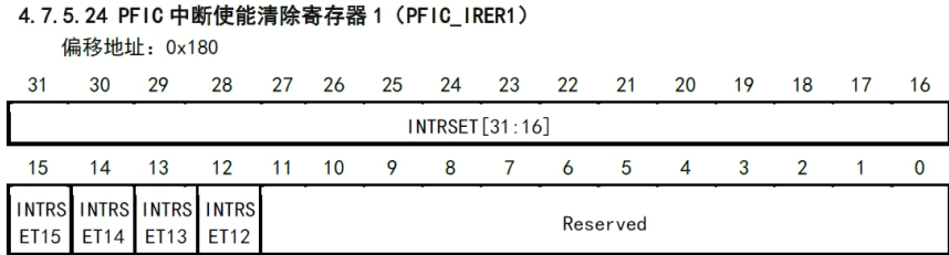
图 1-3 中断使能清除寄存器
