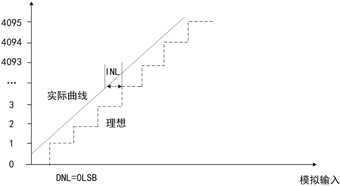
图 1-1-5 ADC 积分误差
