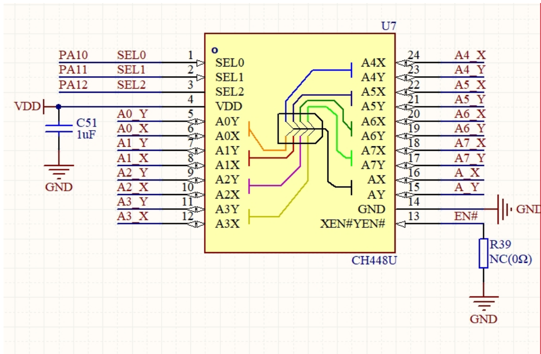
图 2-3CH448 示意图
