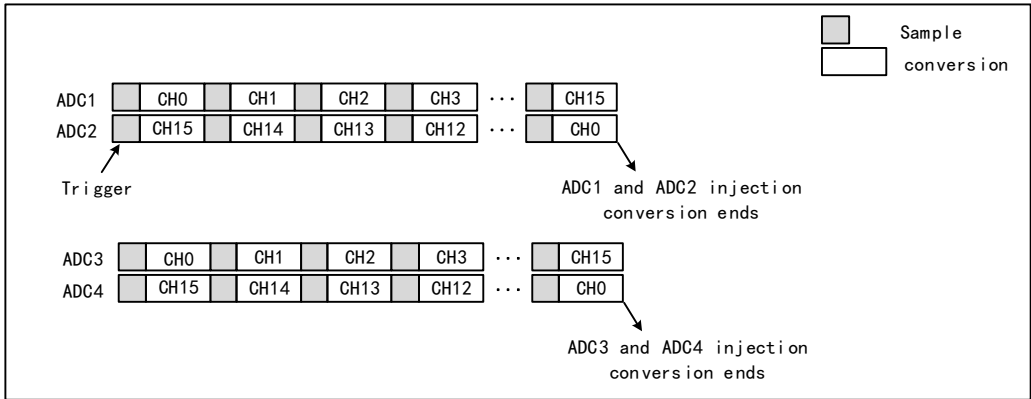
图 1-1 4 组 ADC 同步采样
