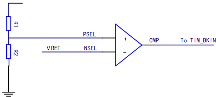
图 2-1 CMP 过流保护拓扑图
