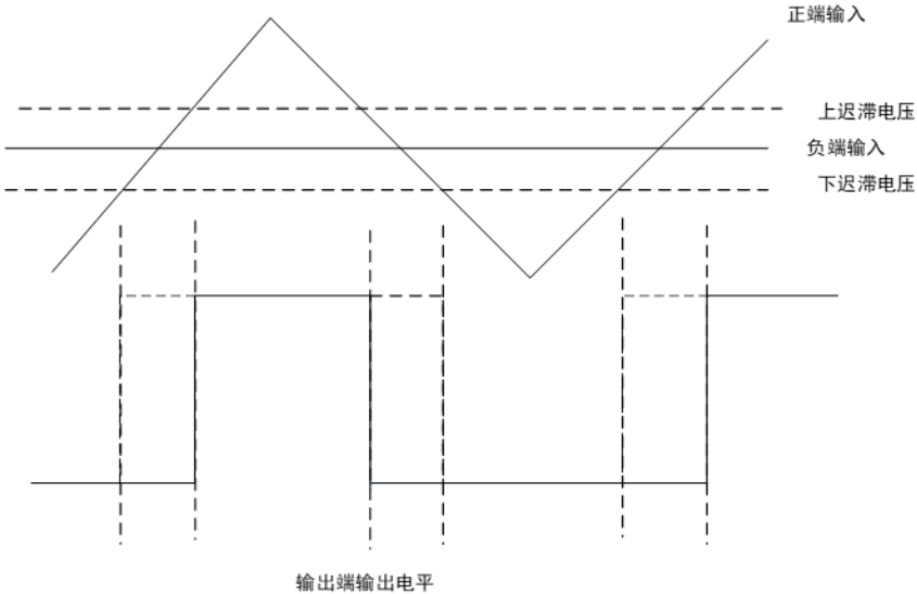
图 1-3 迟滞输出结果
