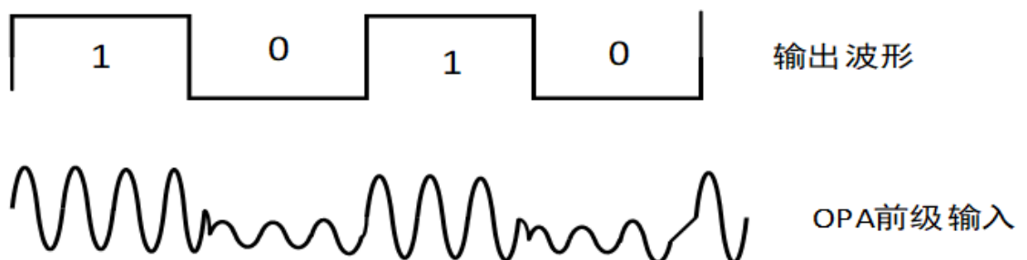
图 2-2 解码结果图
