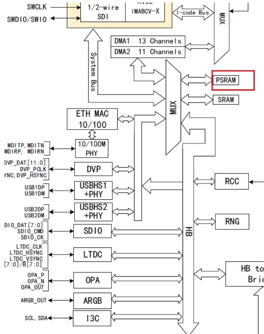
图 1-1 PSRAM 框架
