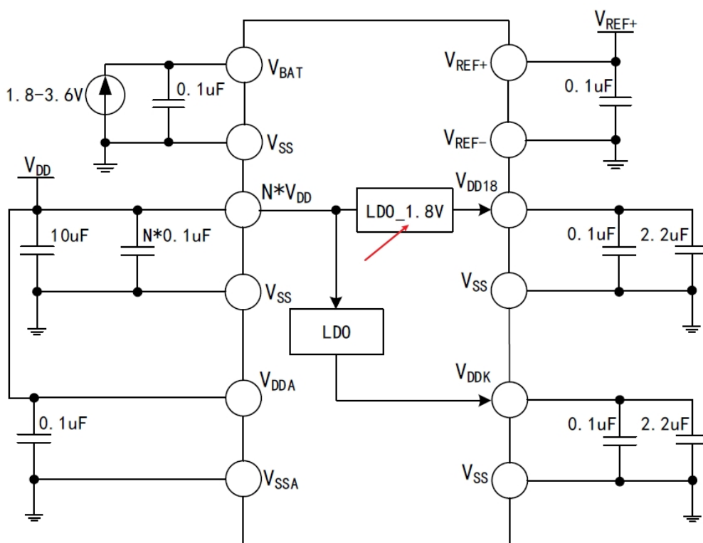
图 1-3 VDD18 框架
