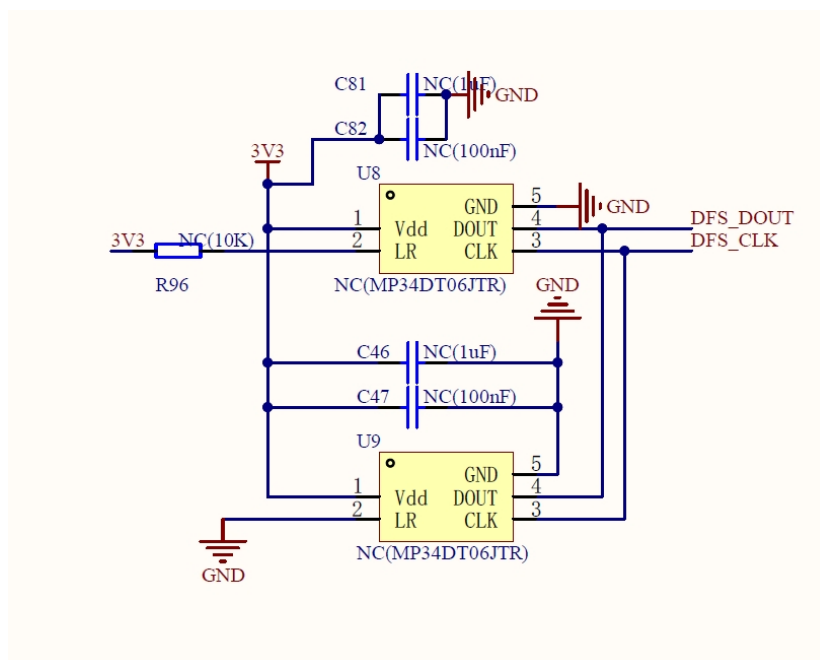
图 2-10 DFSDM 接口麦克风示意图
