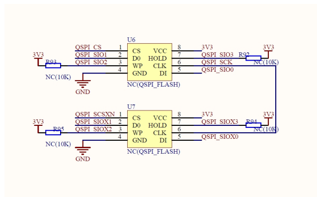
图 2-3 QSPI FLASH 示意图
