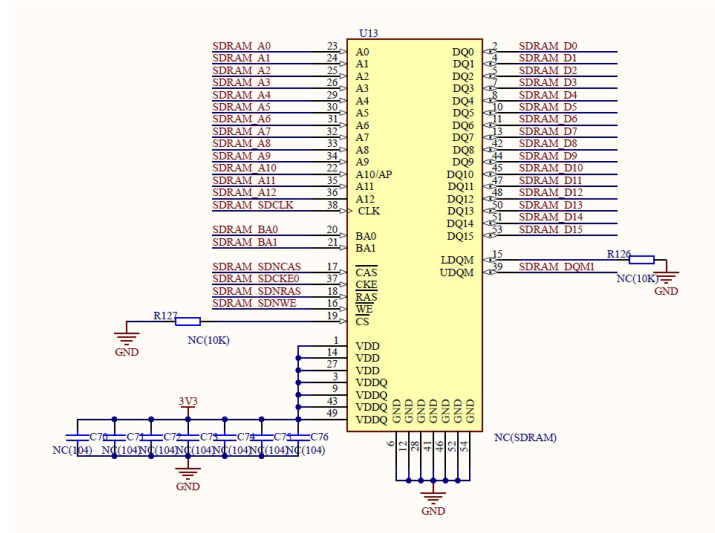
图 2-2 SDRAM 示意图
