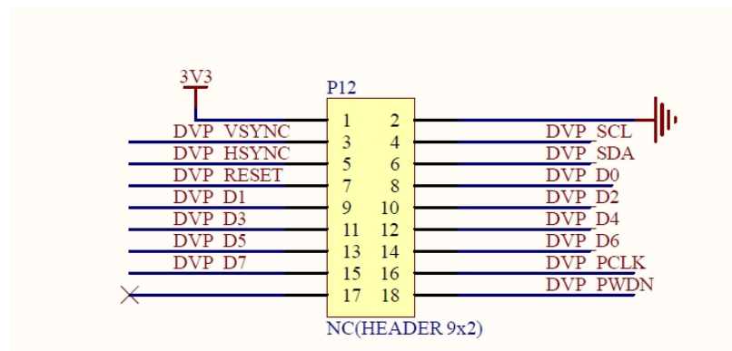
图 2-8 DVP 接口示意图
