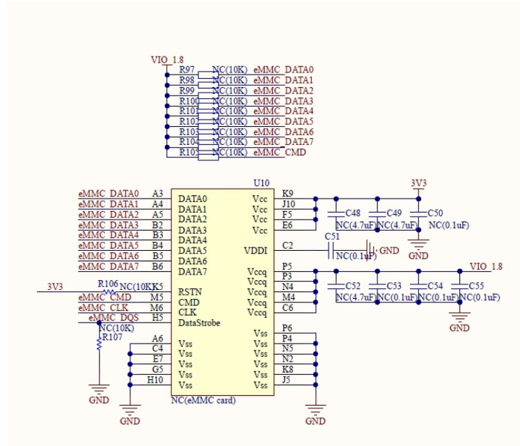
图 2-2 eMMC 示意图
