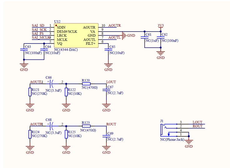
图 2-7 SAI 接口示意图
