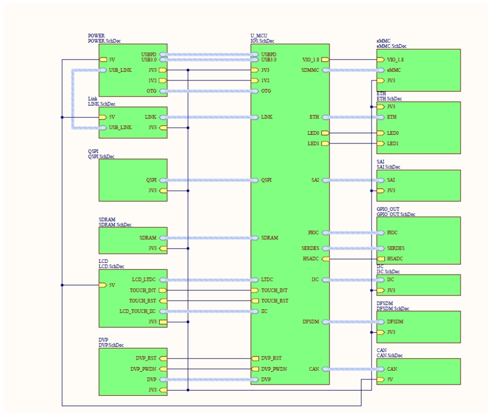
图 2-1 硬件框图
