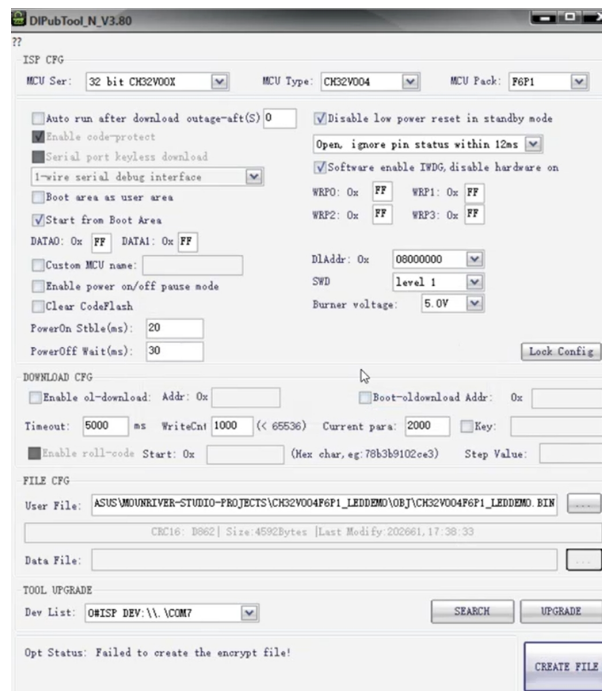
图 2-3 DIPubTool_N_VX.xx.exe 提示
