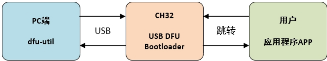
图 2-1 总体结构图
