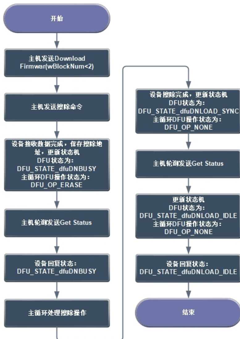
图 2-4 擦除流程
