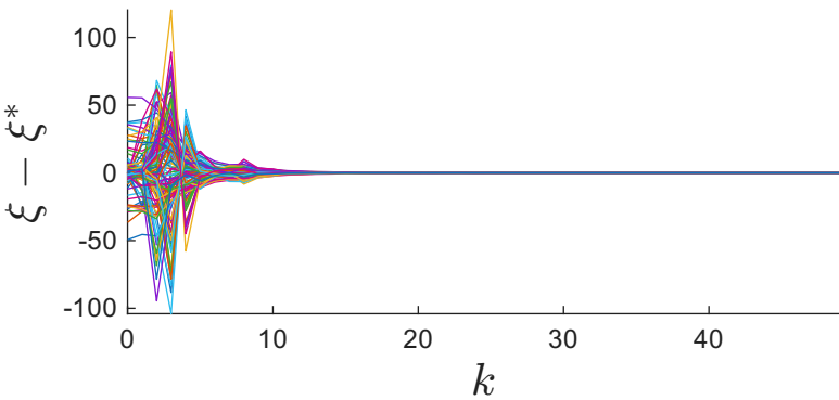
State (Controller) Error
