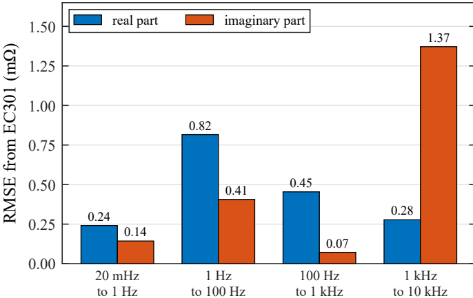
(a) Samsung INR18650-35E
