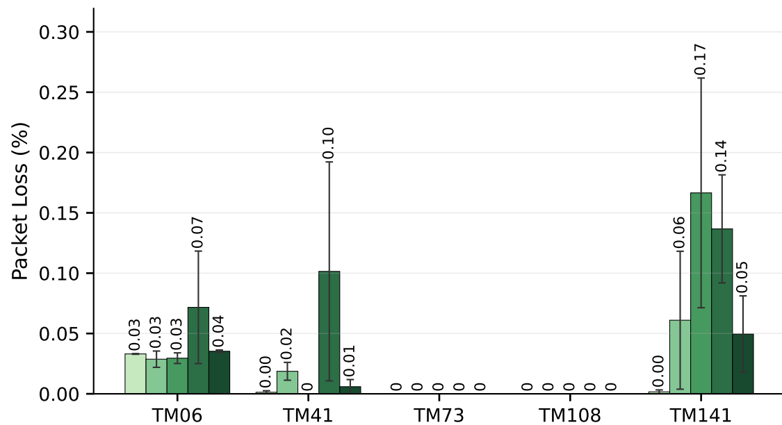
(d) Average Packet Loss ↓
