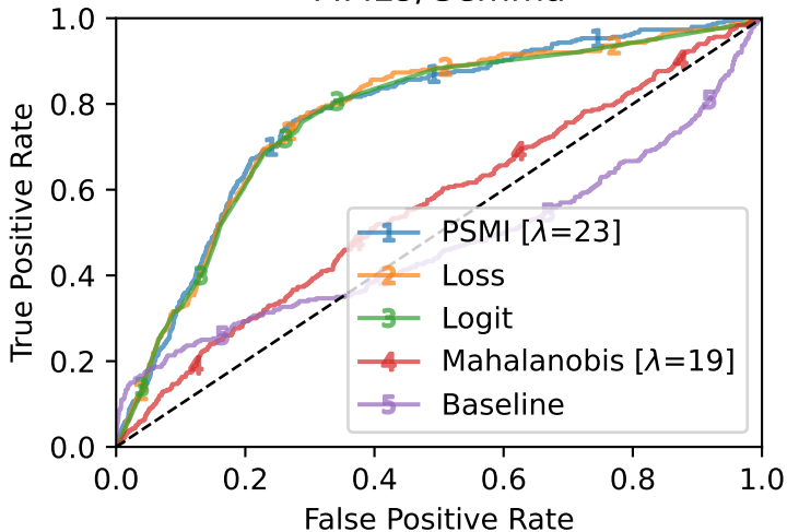
MMLU/Gemma
