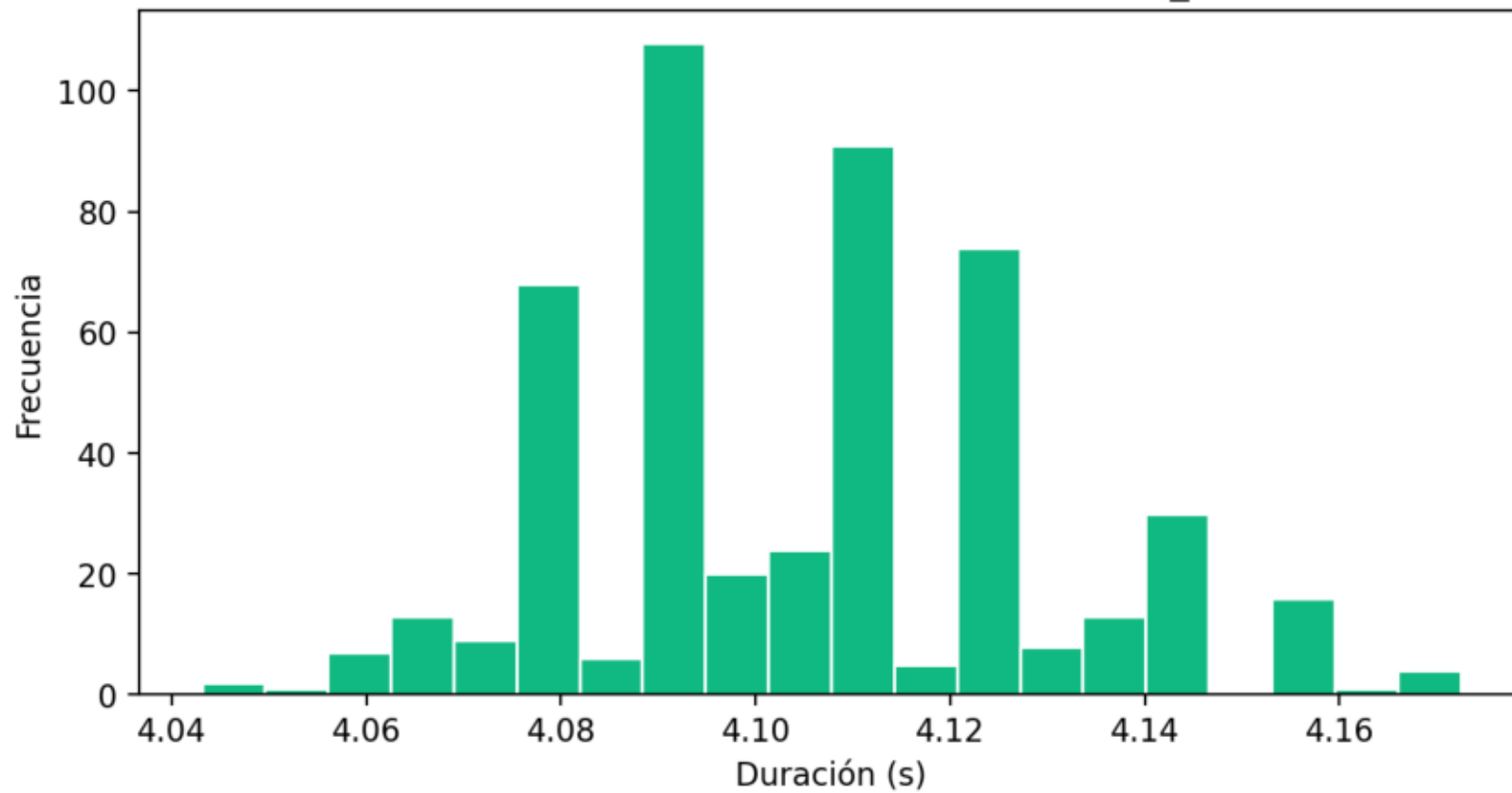
Distribución de latencias - unauthorized_uid
