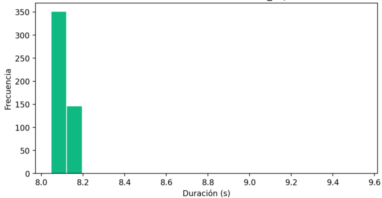
Distribución de latencias - session_expired
