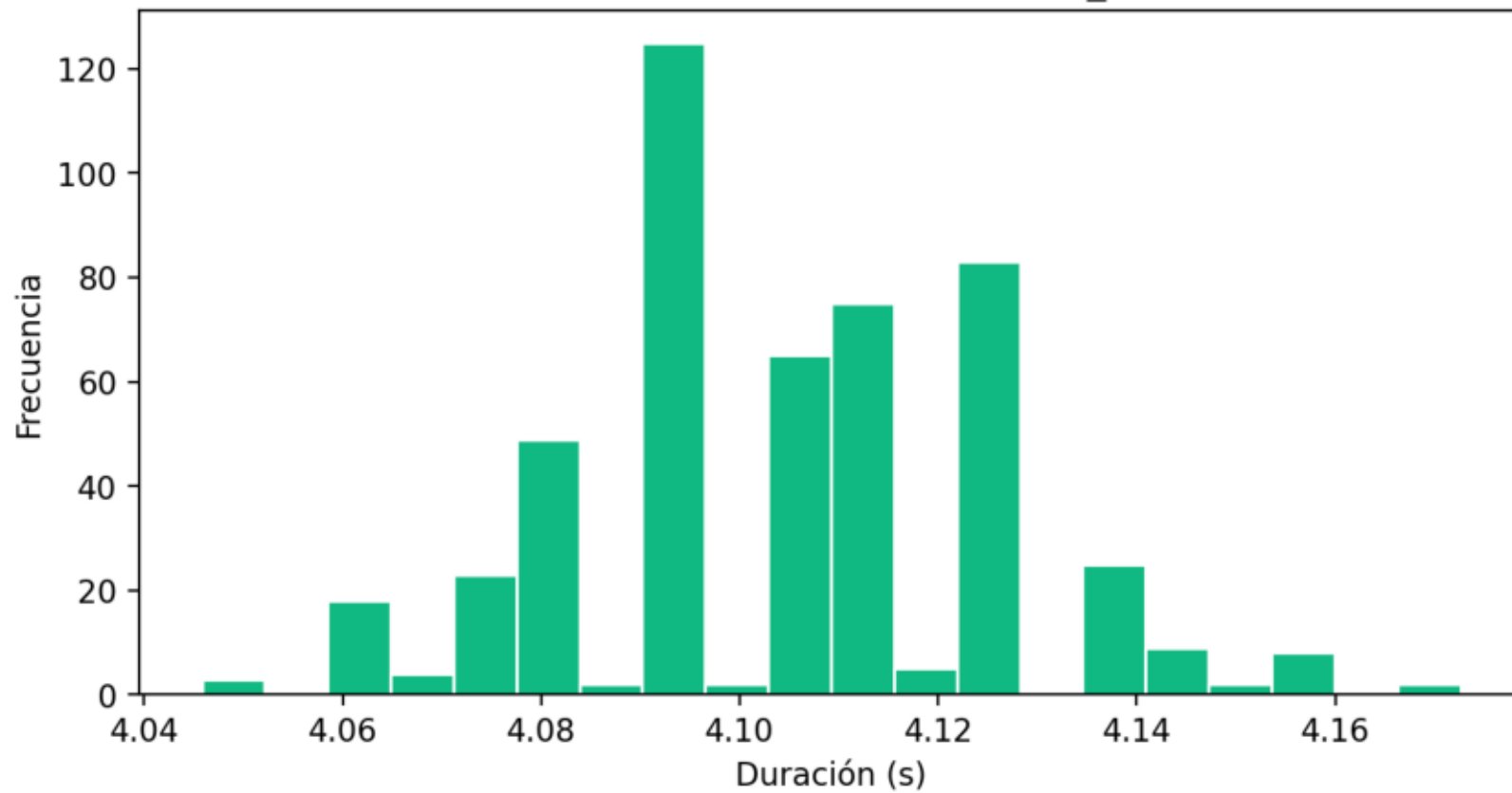
Distribución de latencias - denied_hmac
