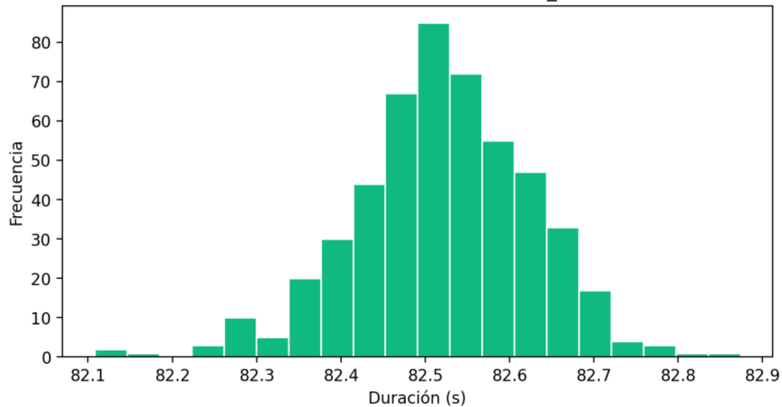
Distribución de latencias - burst_load
