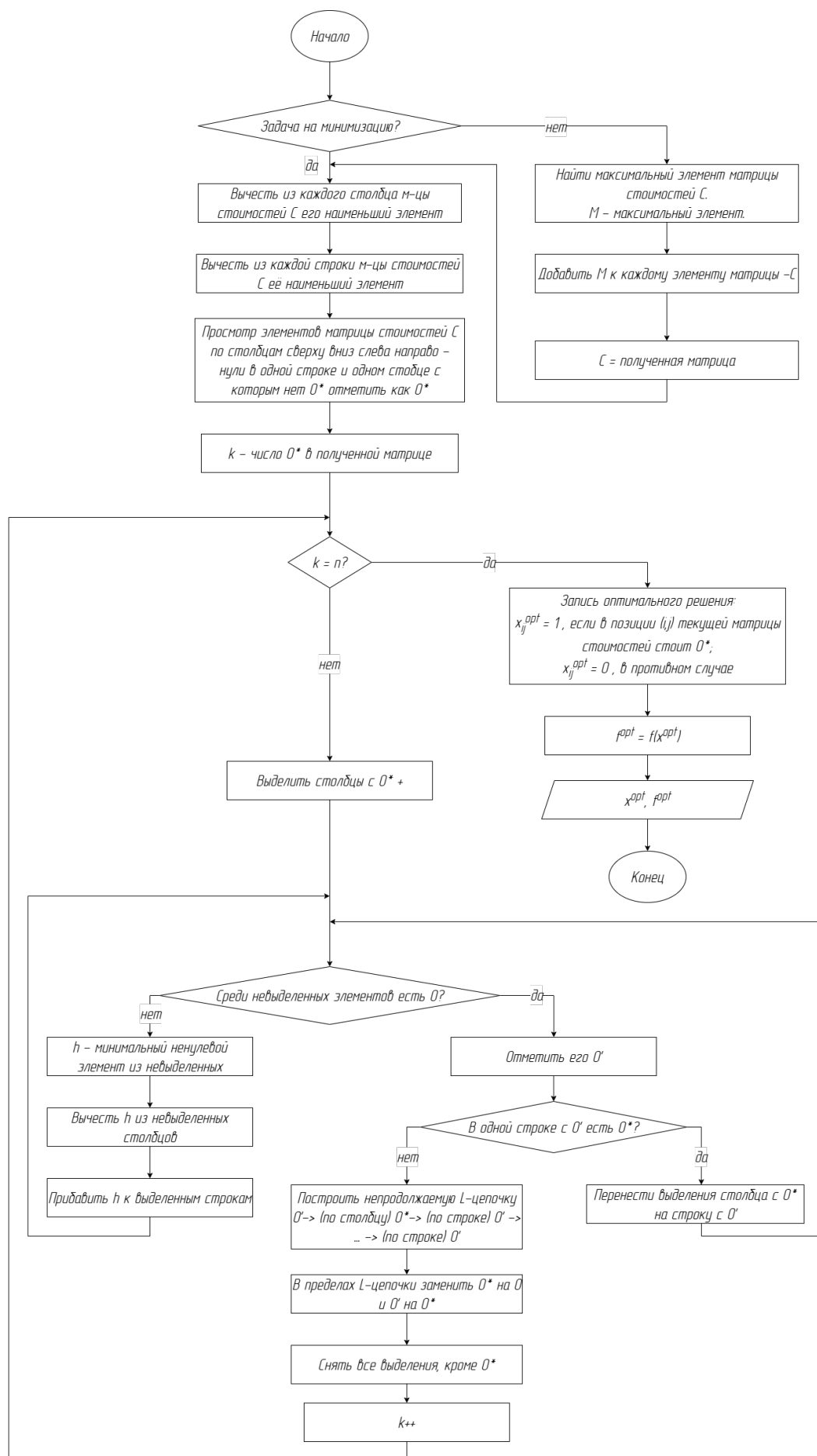
Рисунок 1.1 – Алгоритм решения задачи о назначениях венгерским методом
