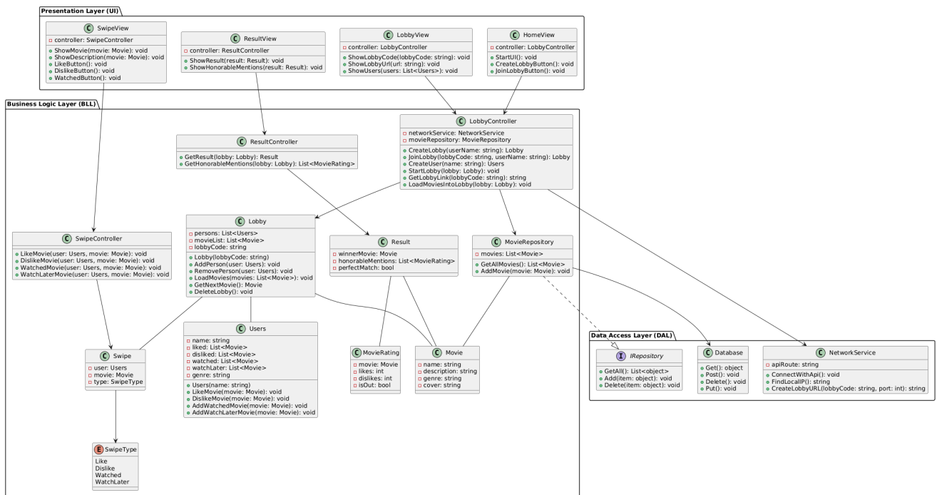
Klassendiagramm - Finnidy
