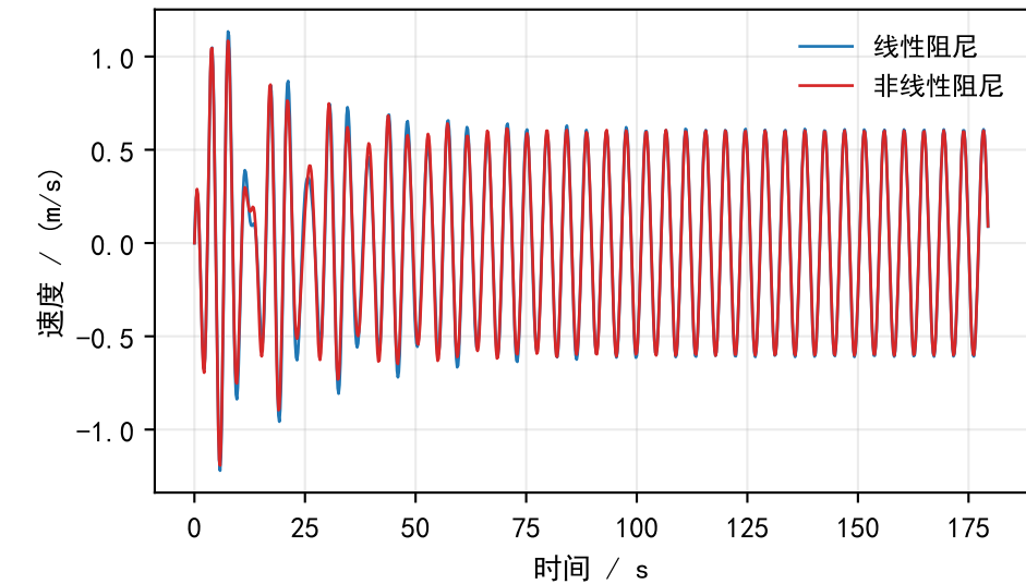
浮子垂荡速度
