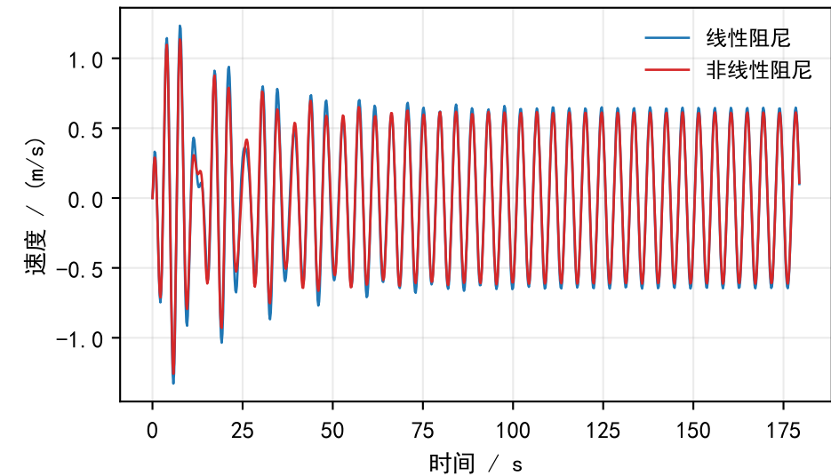
振子垂荡速度
