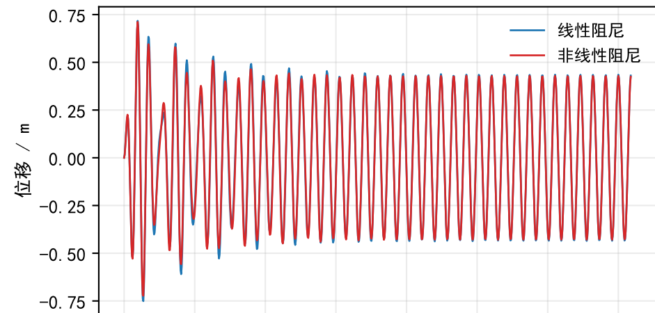
浮子垂荡位移
