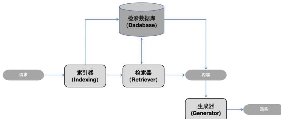
图1 RAG架构
