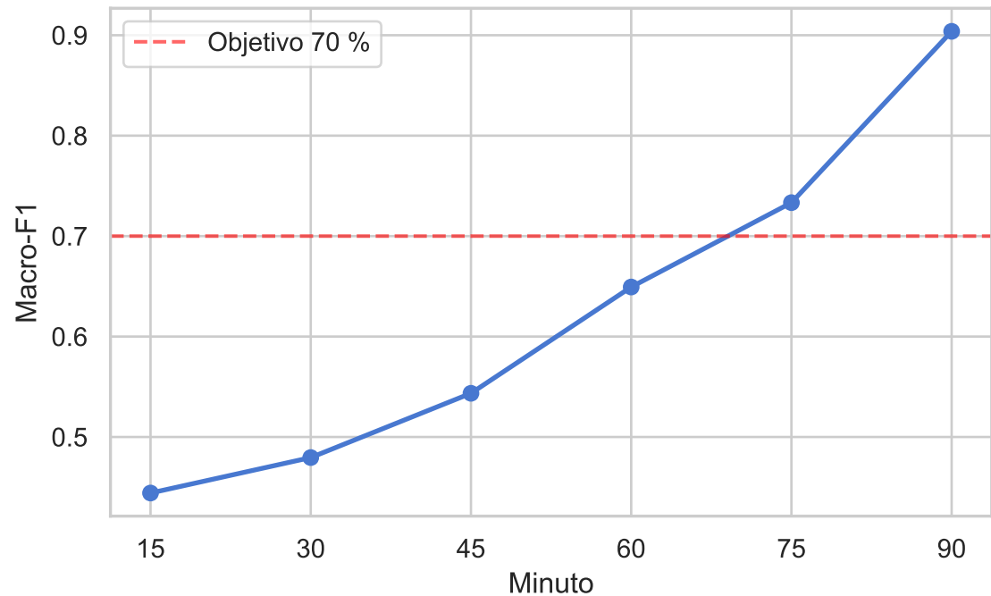
Macro-F1 por minuto — Random Forest
