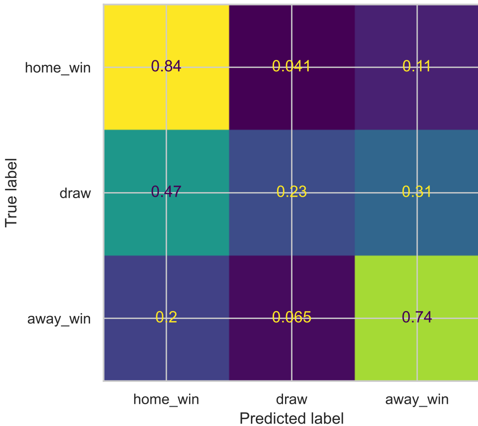
Matriz de confusion normalizada — Random Forest
