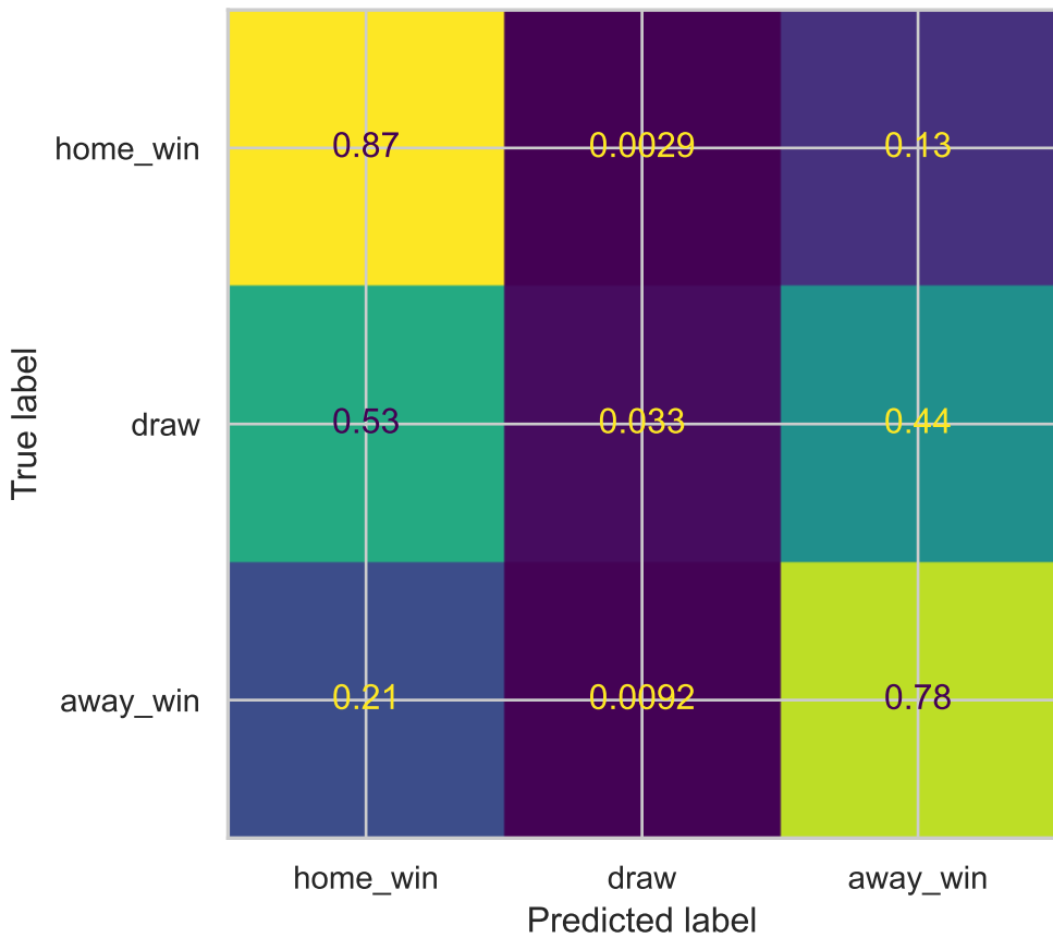
Matriz de confusion normalizada — SVM lineal
