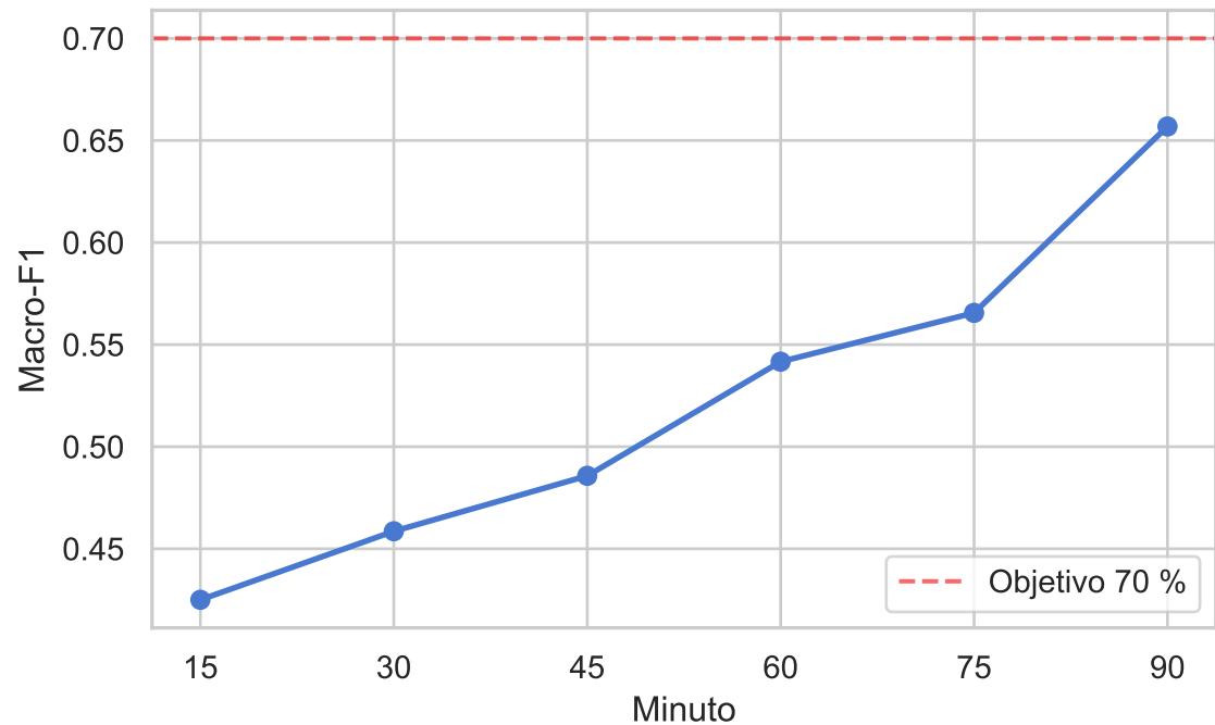
Macro-F1 por minuto — SVM lineal
