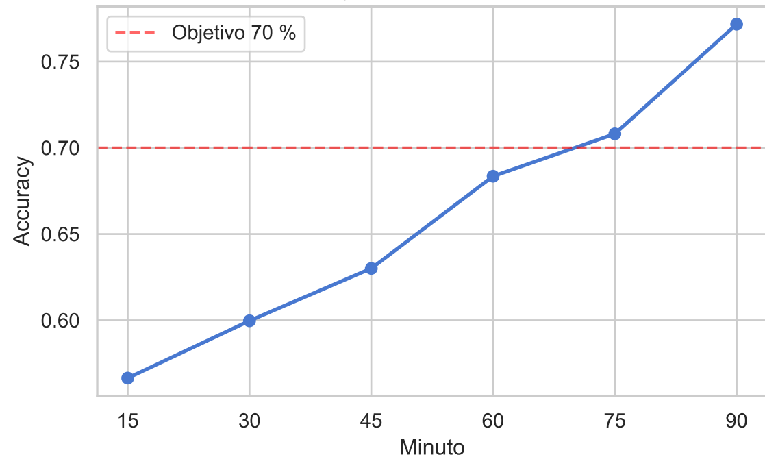
Accuracy por minuto — SVM lineal
