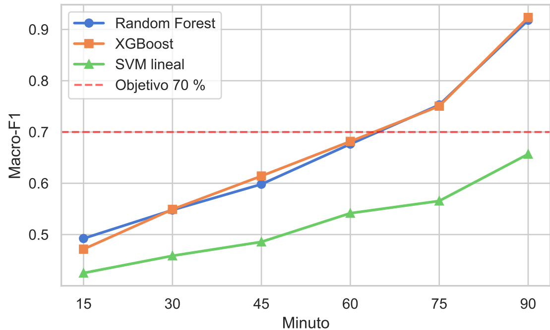
Macro-F1 por minuto — Comparación de modelos
