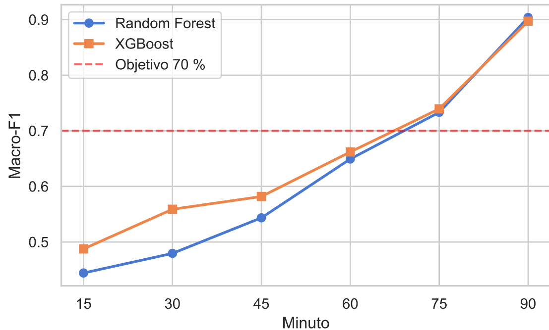
Macro-F1 por minuto — RF vs XGBoost
