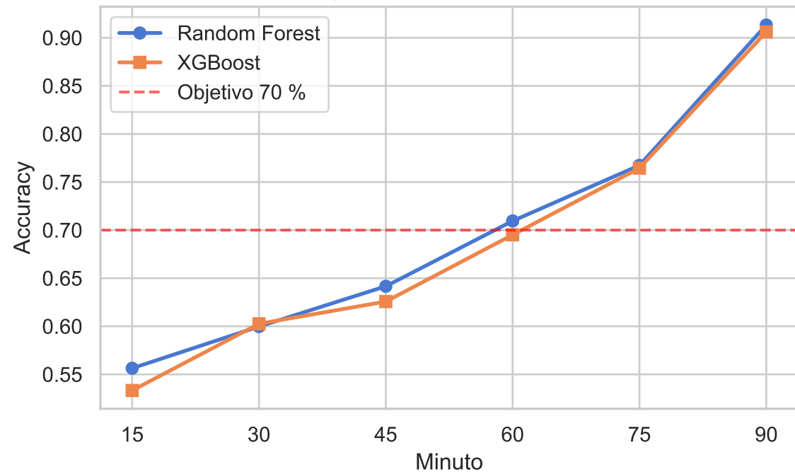
Accuracy por minuto — RF vs XGBoost
