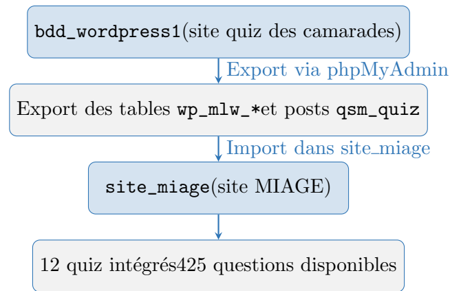
FIGURE 2 – Schéma de la fusion des bases de données
