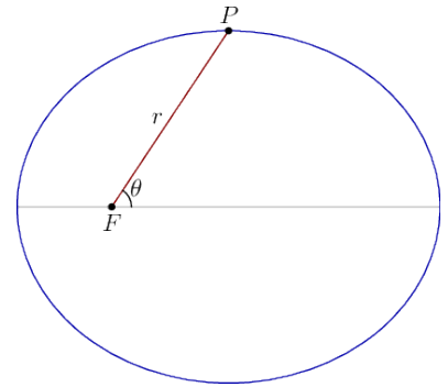
Trascuriamo il moto del Sole considerandolo fermo.
