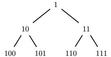
Figura 1: I primi tre livelli dell'albero che contiene \mathbb{N}^+ in base 2
