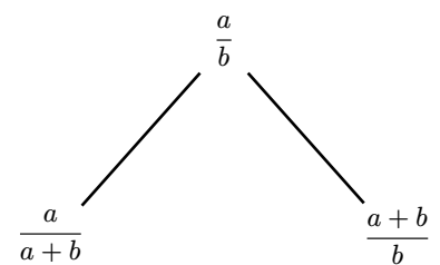
Figura 15: Rappresentazione visuale di \mathcal{D} e \mathcal{S} .
