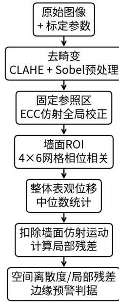
图 1 优化后的墙面图像检测与边缘预警算法流程
