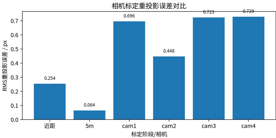
图 2 各标定阶段及四台相机的 RMS 重投影误差
