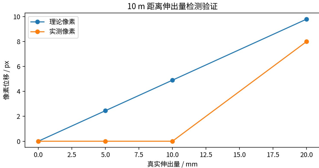
图 3 10 m 距离下伸出量理论像素与实测像素对比
