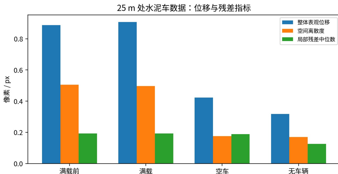
图 5 25 m 处水泥车数据的整体位移、空间离散度与局部残差
