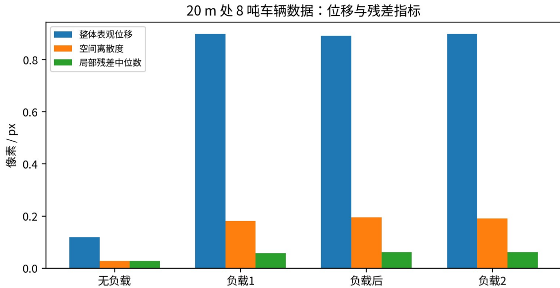
图 4 20 m 处 8 吨车辆数据的整体位移、空间离散度与局部残差
