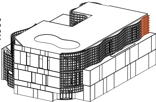
AXONOMETRY 1:500
