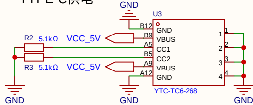
TYPE-C供电
