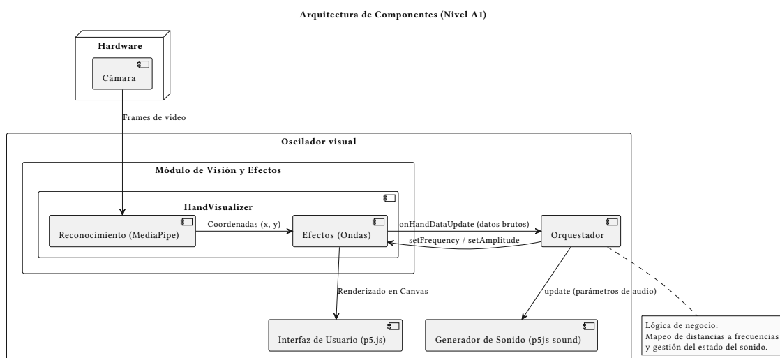
Figura 2: Arquitectura de componentes del sistema (Nivel A1).
