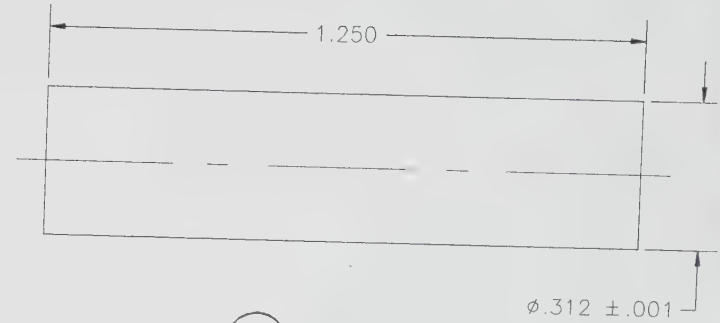
(23) PIVOT PIN
