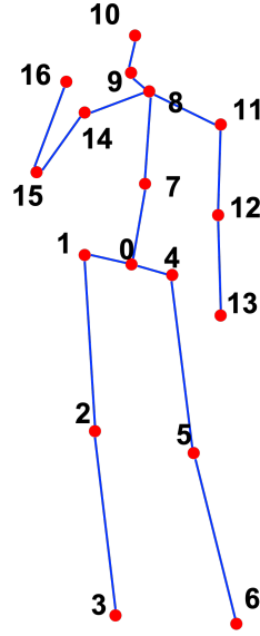
Рис. 13: Схема трехмерной позы в формате Human3.6М
