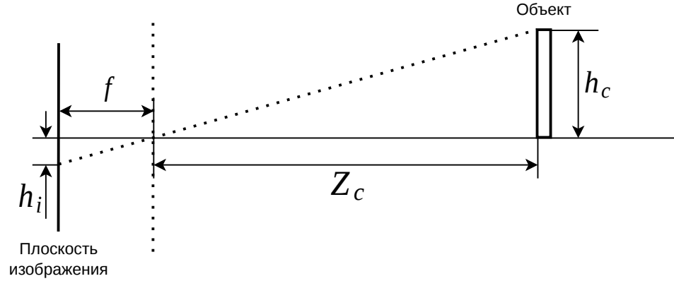
Рис. 4: Простейшая модель камеры-обскуры.
