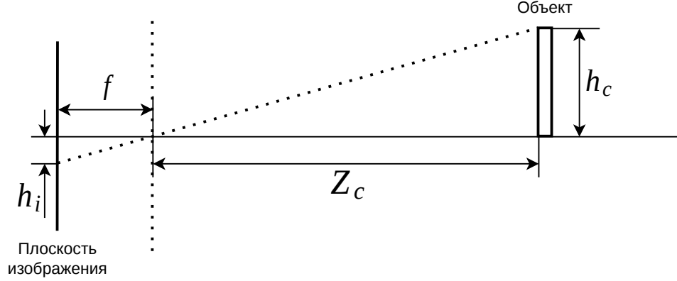
Рис. 3: Простейшая модель камеры-обскуры
