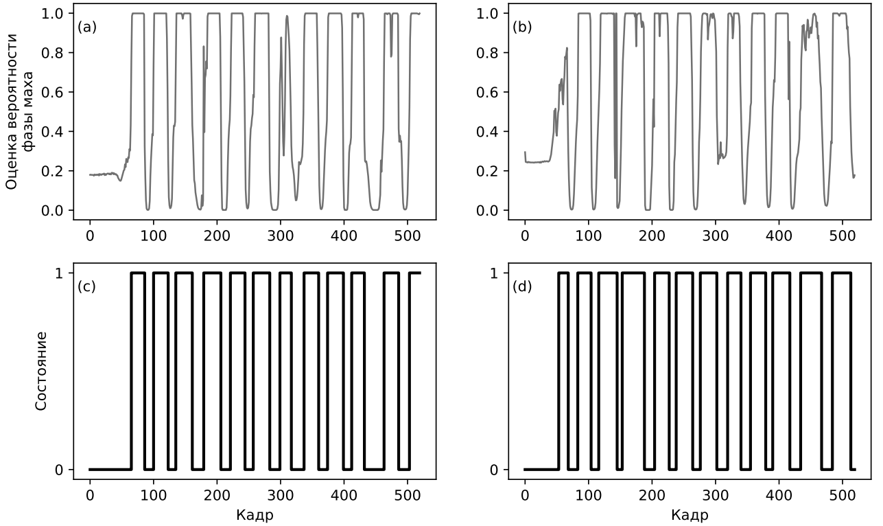
Рис. 5: Результат сегментации фаз походки на видео 2. (a) Вероятности фазы маха для правой ноги; (b) Вероятности фазы маха для левой ноги; (c) Восстановленная последовательность состояний для правой ноги; (d) Восстановленная последовательность состояний для левой ноги.
