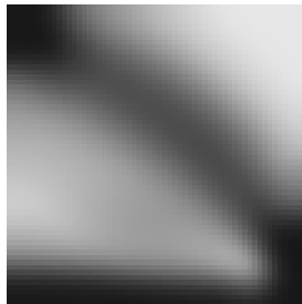
Iteración 200 — Flexibilidad 29.73
