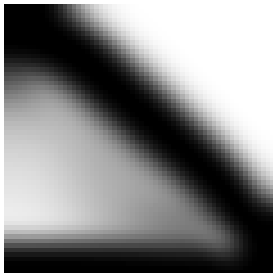
Iteración 5 — Flexibilidad 33.61
