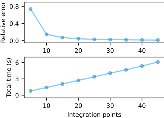
BEM
