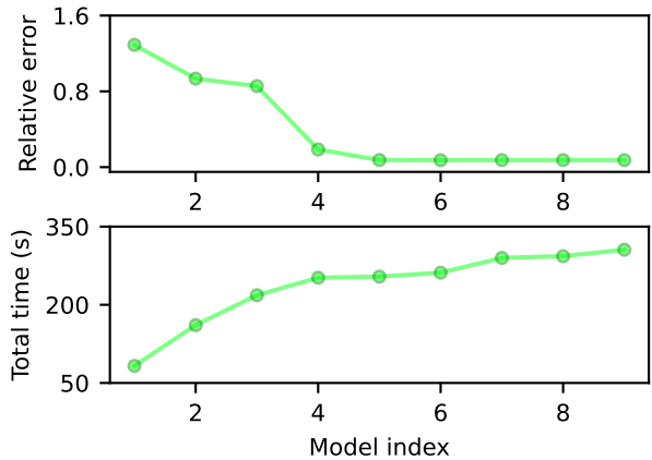
PINN
