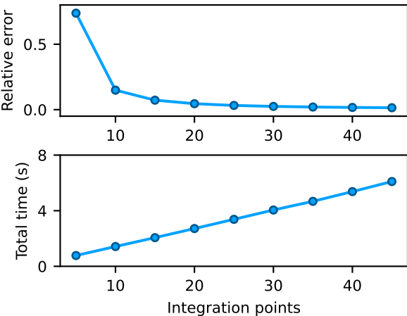
BEM
