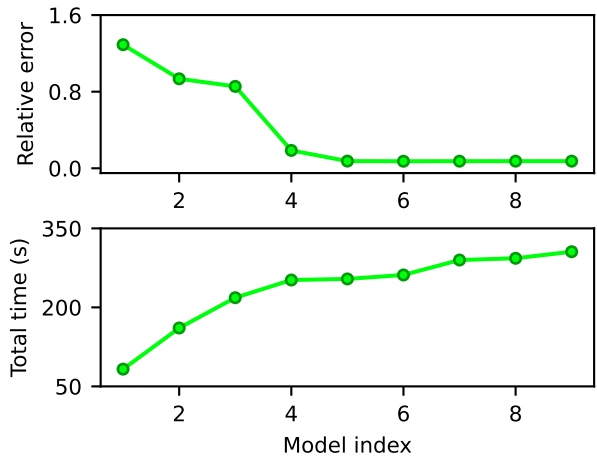
PINN
